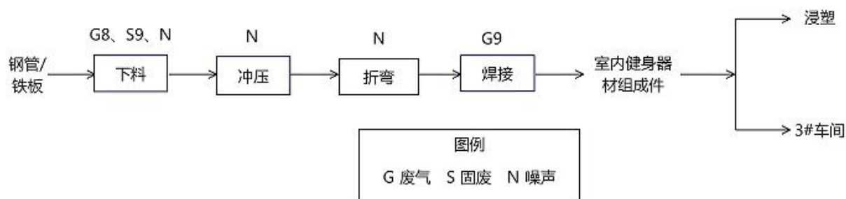
图 2-4 2#生产车间机加工工艺流程及排污节点图
