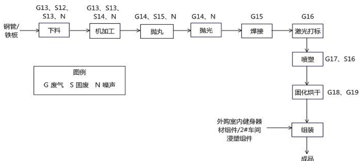
图 2-5 3#生产车间工艺流程及排污节点图
