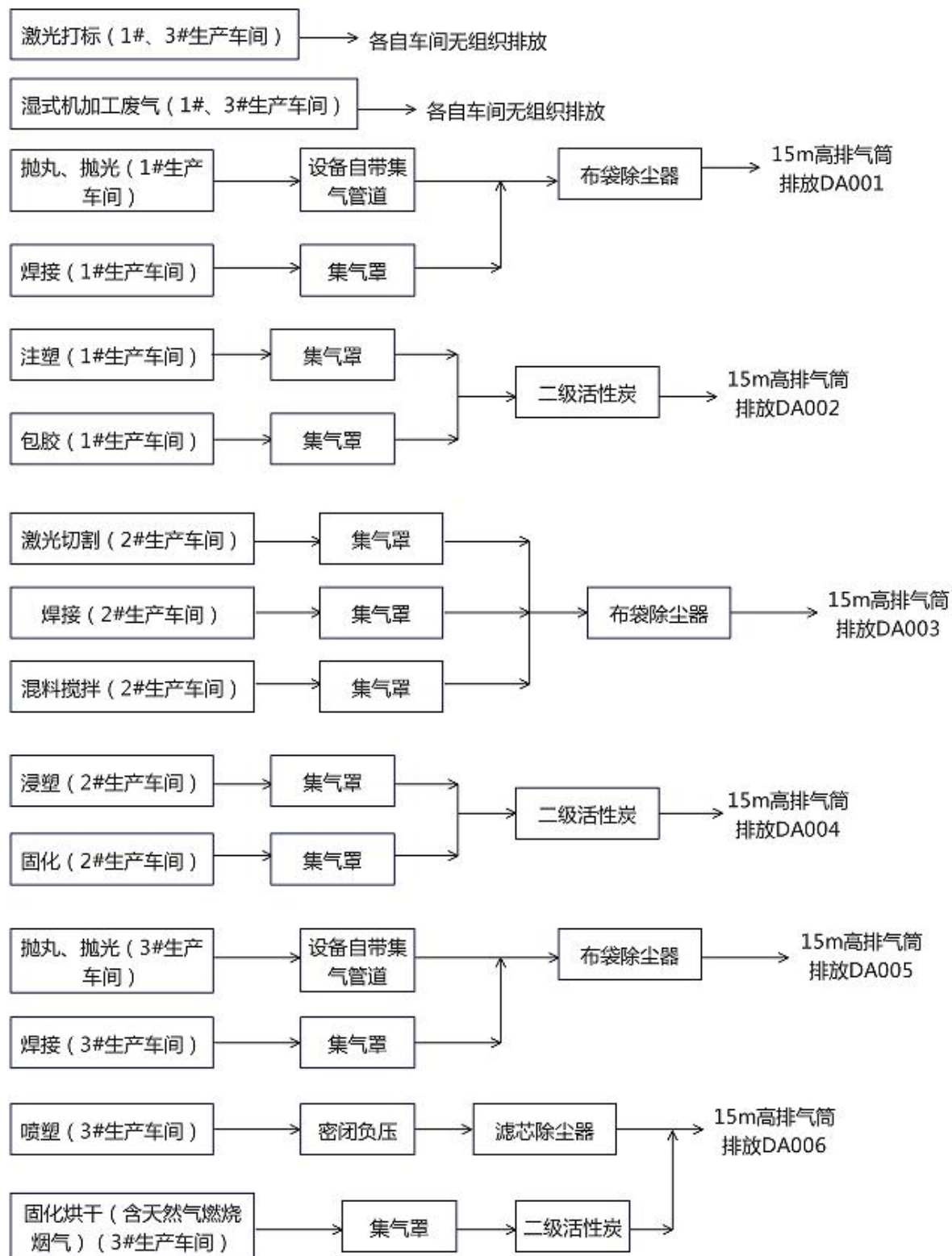
图 4-1 废气收集治理排放示意图
