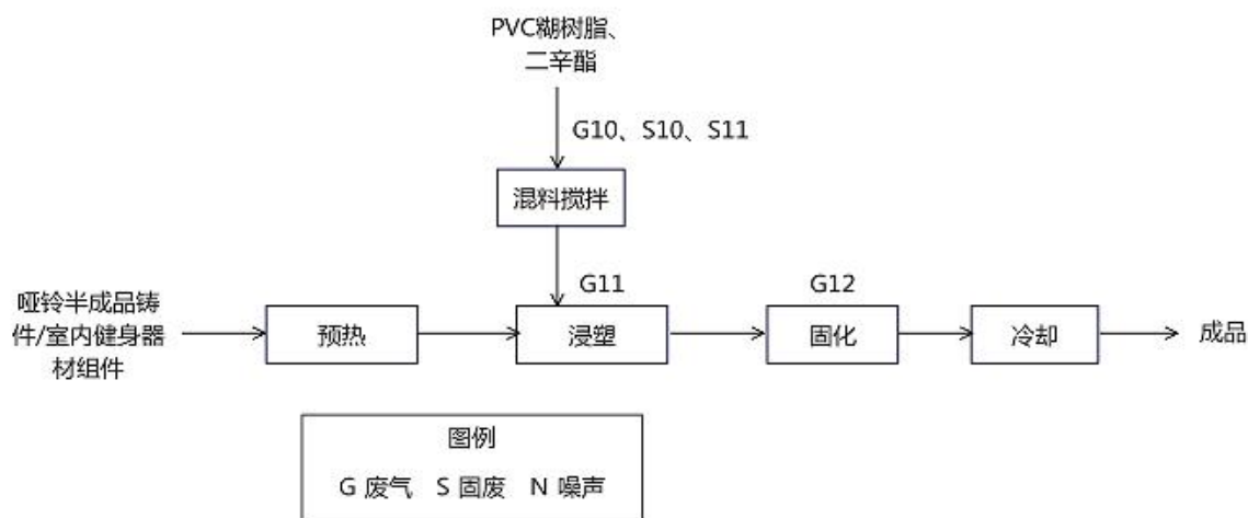
图 2-5 2#生产车间浸塑工艺流程及排污节点图
