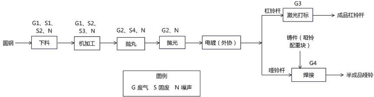
图 2-2 1#生产车间机加工工艺流程及排污节点图
