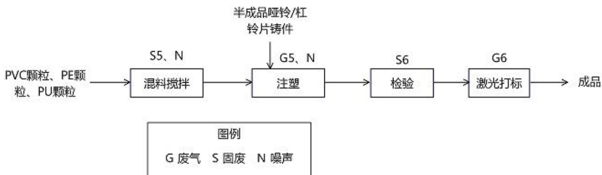
图 2-3 1#生产车间注塑工艺流程及排污节点图
