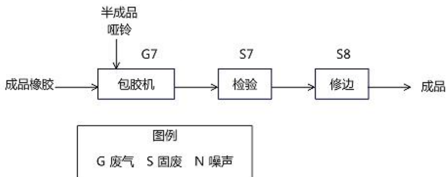
图 2-3 1#生产车间包胶工艺流程及排污节点图
