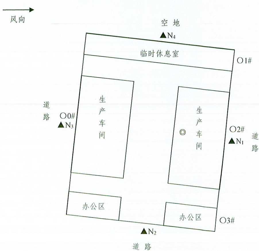
附图：检测点位布设示意图
