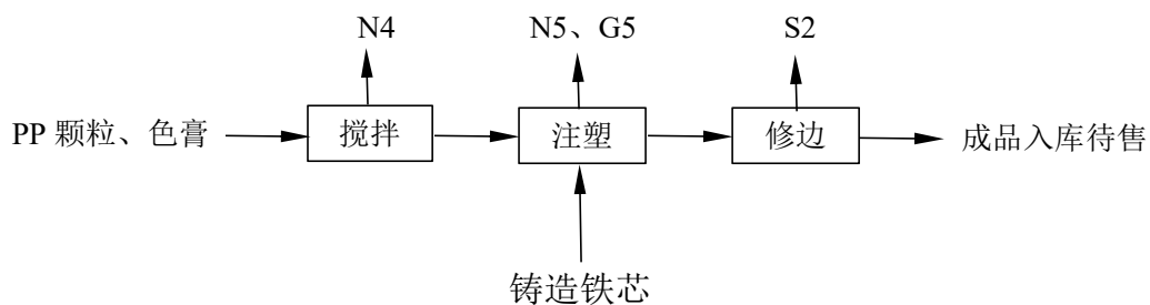
图 2-4 注塑生产工艺流程及排污节点图
