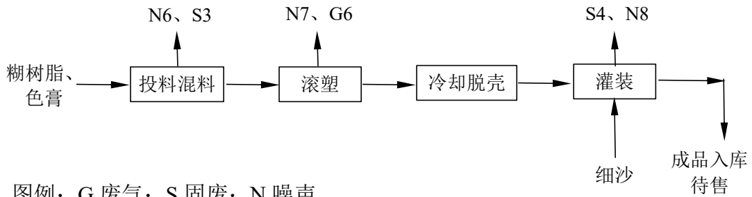
图 2-5 滚塑生产工艺流程及排污节点图
