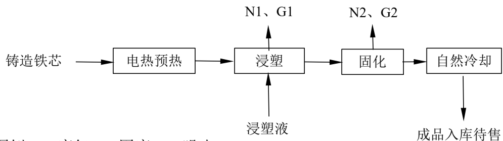
图 2-2 浸塑生产工艺流程及产污节点图
