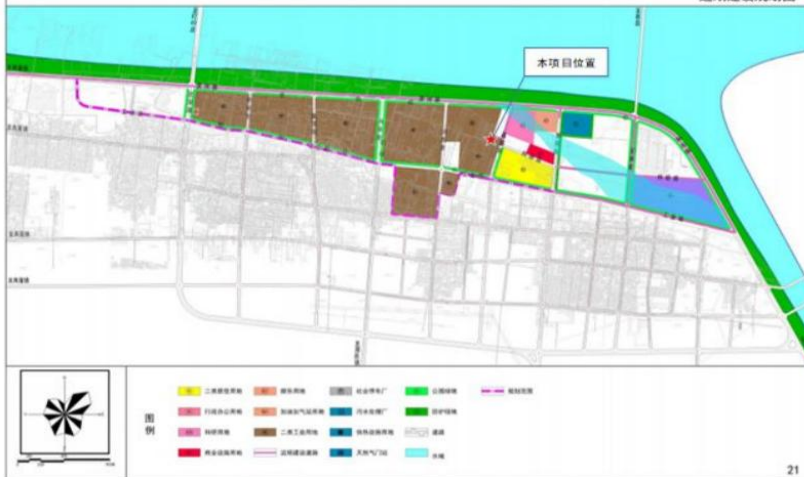
附图 4 园区用地布局规划图
