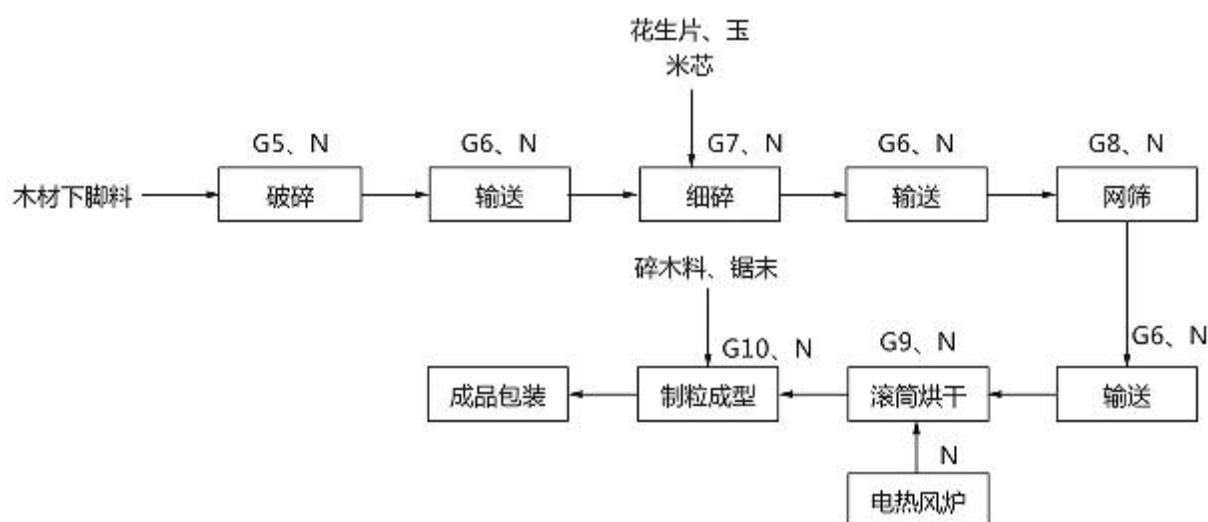
图 2-3 生物质颗粒生产工艺流程及排污节点图
