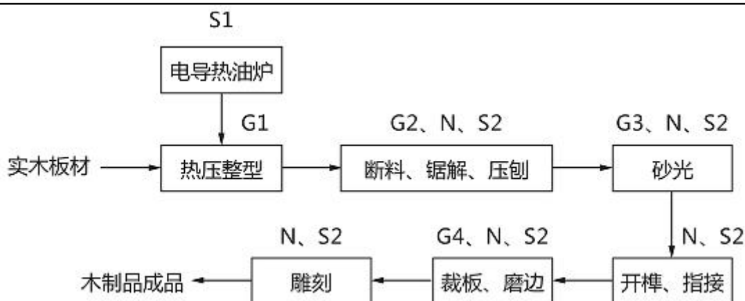
图 2-2 木制品生产工艺流程及排污节点图
