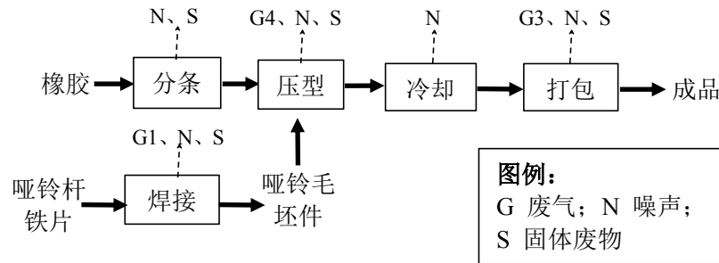
图 5 橡胶哑铃生产工艺流程图
