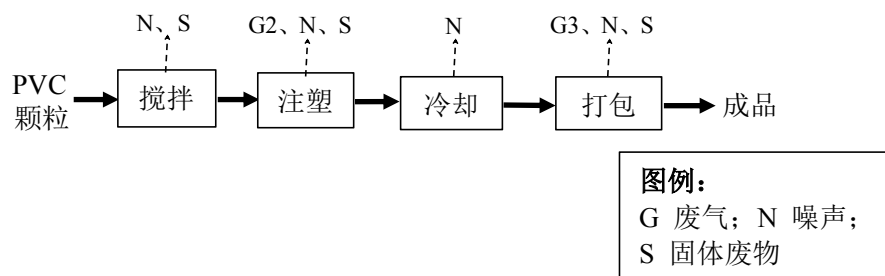
图 8 纺织配件生产工艺流程图
