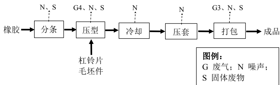
图 7 橡胶杠铃片生产工艺流程图
