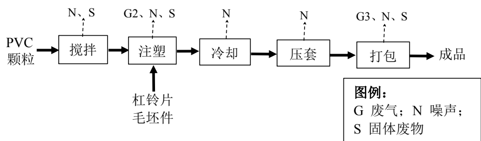
图 6 塑料杠铃片生产工艺流程图
