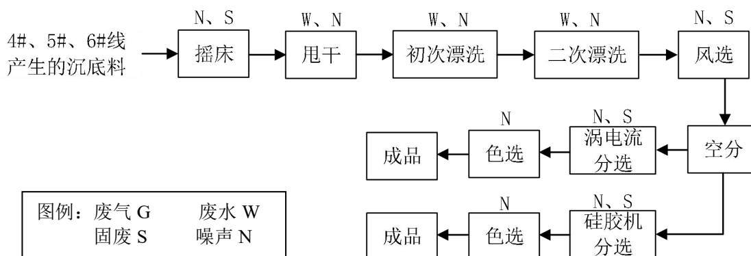
图 2-6 7#线生产工艺流程图
