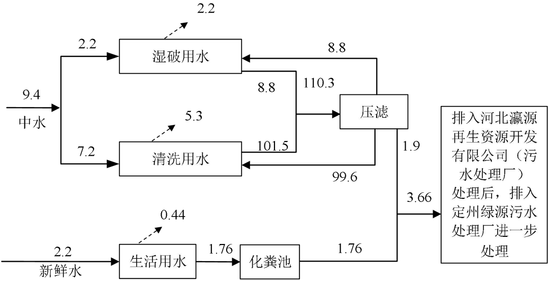
图2-1 项目水平衡图 单位：m 3 /d（虚线箭头为损耗水量）
