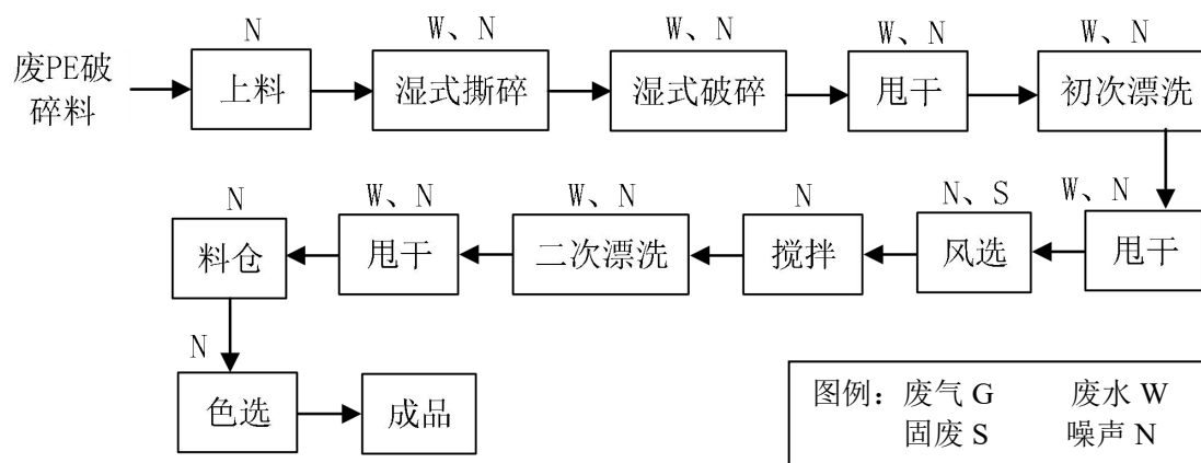
图 2-3 4#线生产工艺流程图
