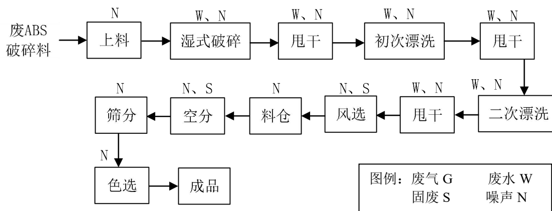
图 2-4 5#线生产工艺流程图
