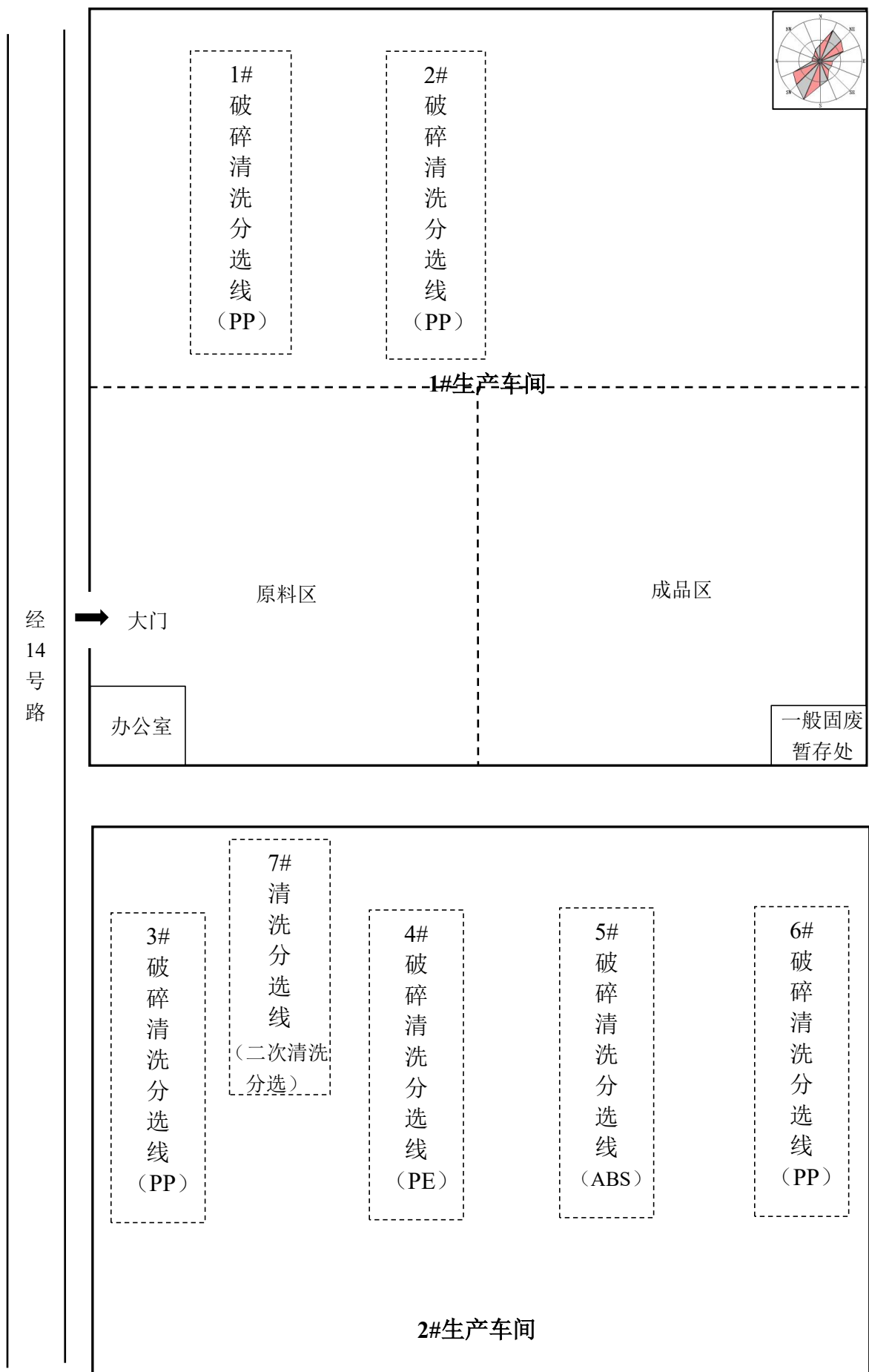
附图3 厂区平面布置示意图 (比例尺 1: 600)
