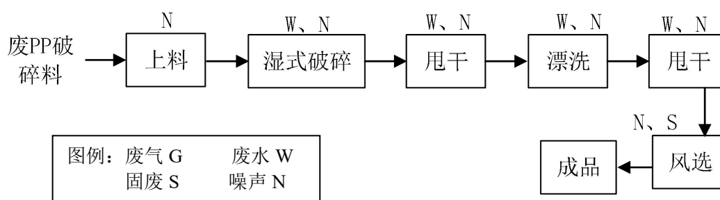
图 2-5 6#线生产工艺流程图
