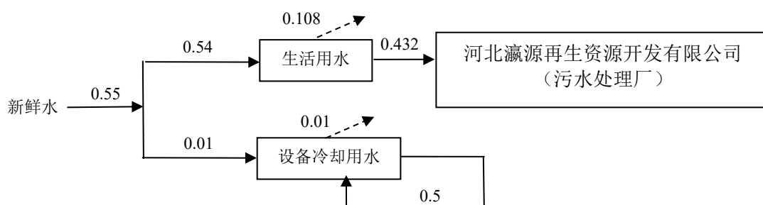
图1 本项目给排水平衡图 单位： \text{m}^3/\text{d}
