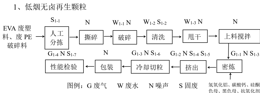
图2 低烟无卤再生颗粒生产工艺流程及排污节点图
