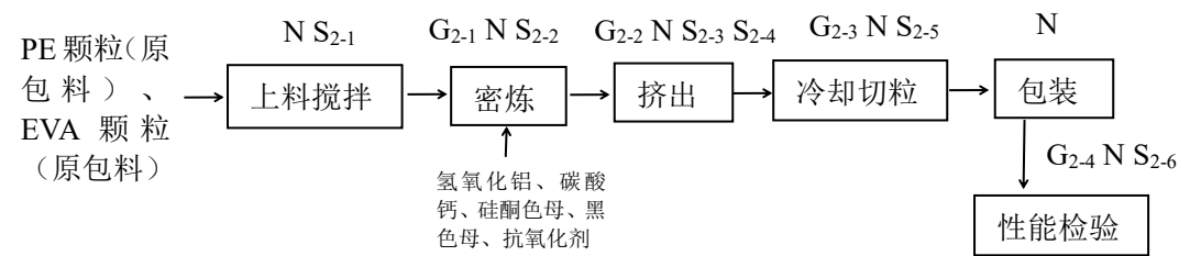
图 3 低烟无卤颗粒生产工艺流程及排污节点图
