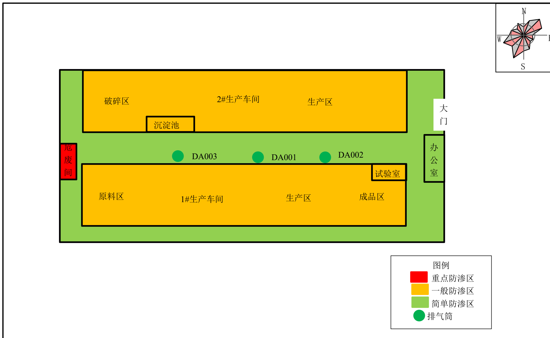
附图 4 厂区平面布置及分区防渗示意图
