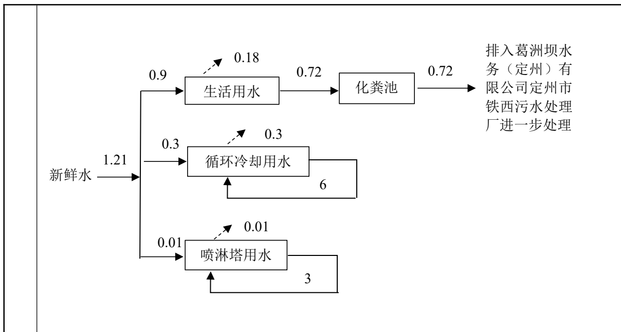
图1 项目给排水平衡图 单位: m 3 /d
