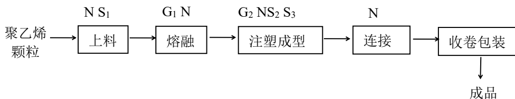
图2 生产工艺流程及排污节点图
