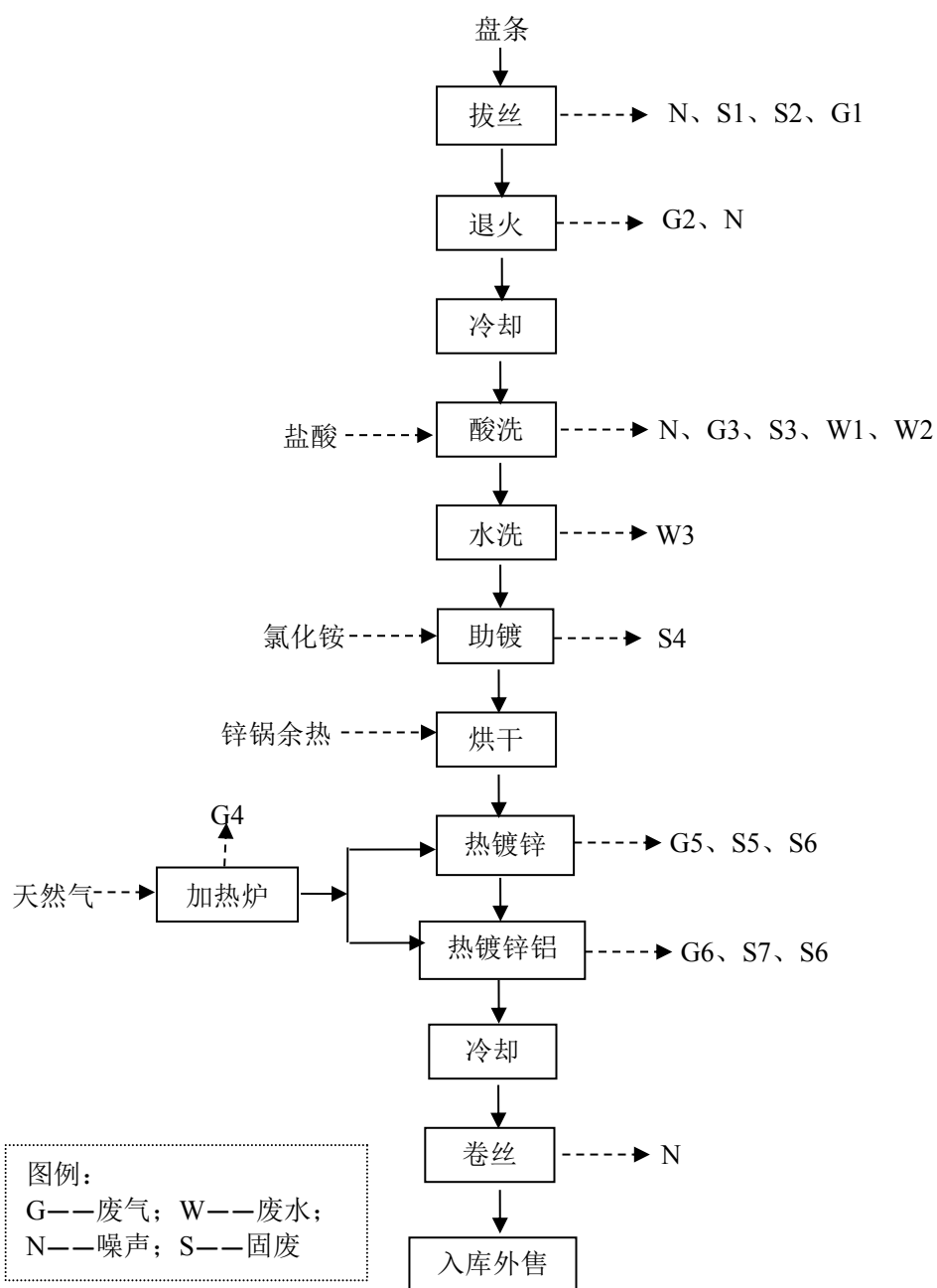
图 2 热镀铝锌丝生产工艺流程及排污节点图
