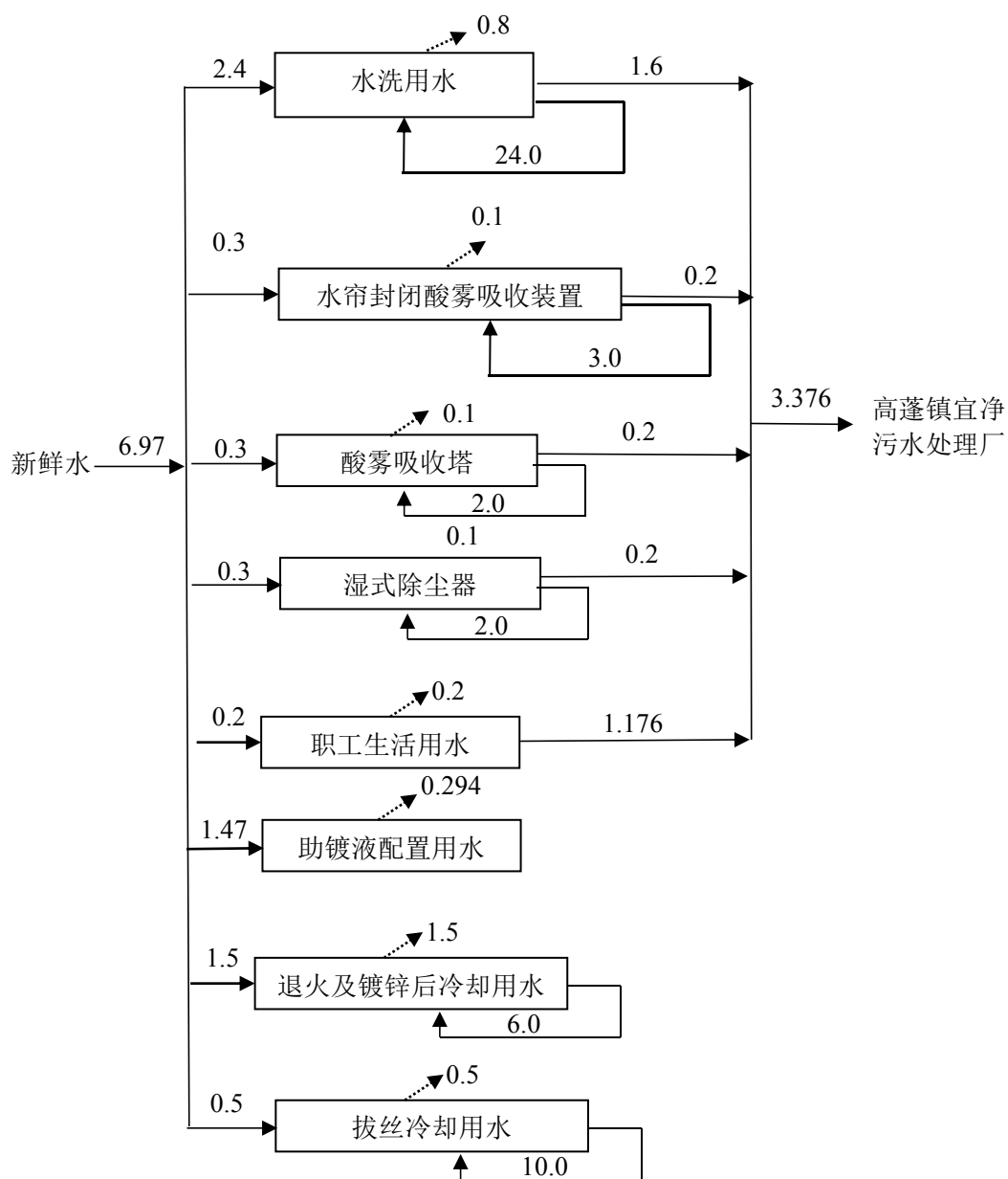
图 1 拟建项目水量平衡图 单位: m³/d
