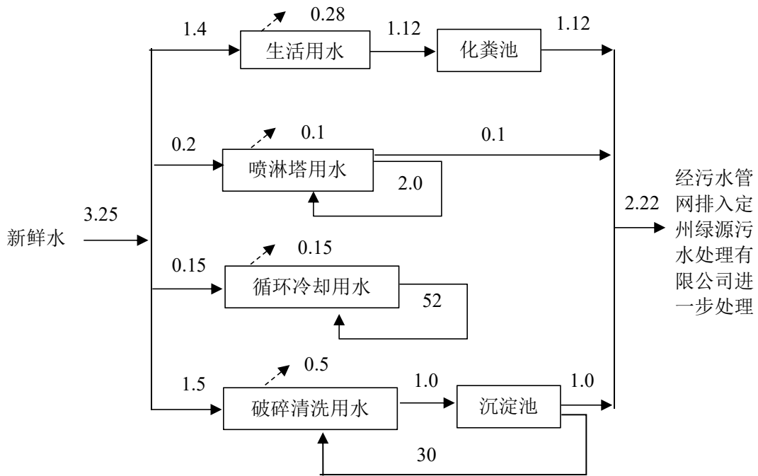
图 2 扩建项目完成后全厂给排水平衡图 单位：m 3 /d
