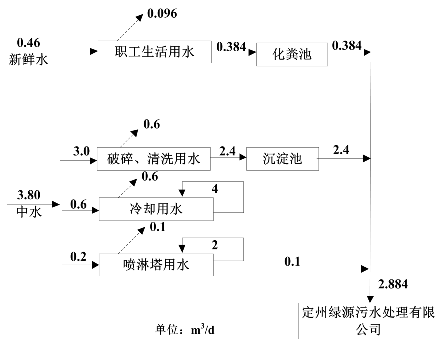
图1 项目给排水平衡图
