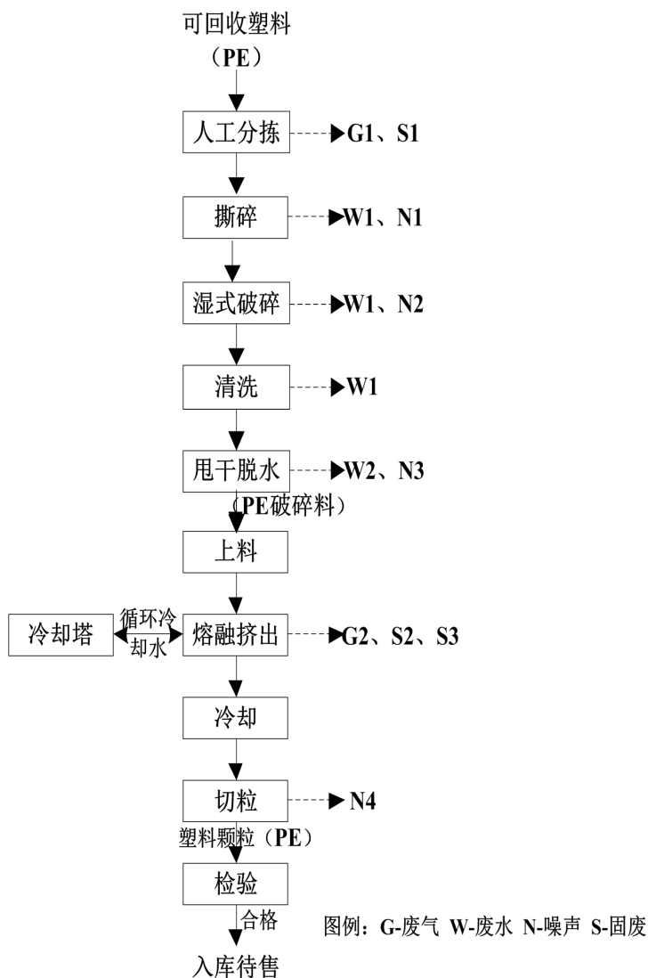
图2 生产工艺流程及产污节点图
