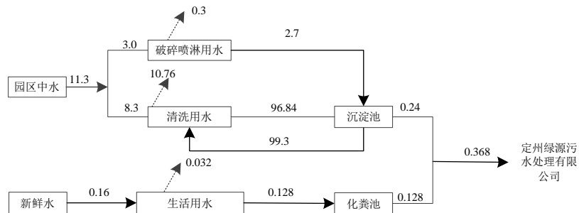
图2-1 项目给排水平衡图 单位：m 3 /d
