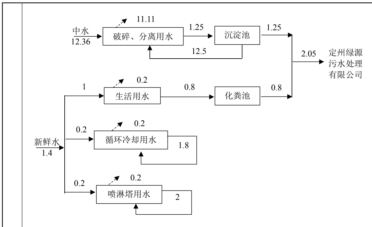
图 1 项目水平衡图 单位: m 3 /d
