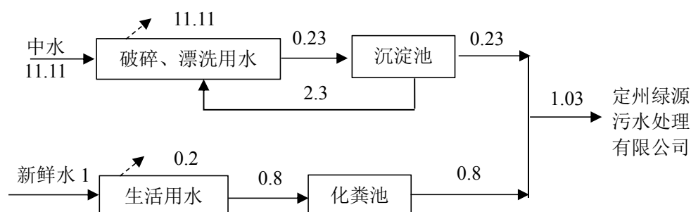
图 1 项目水平衡图 单位： \text{m}^3/\text{d}
