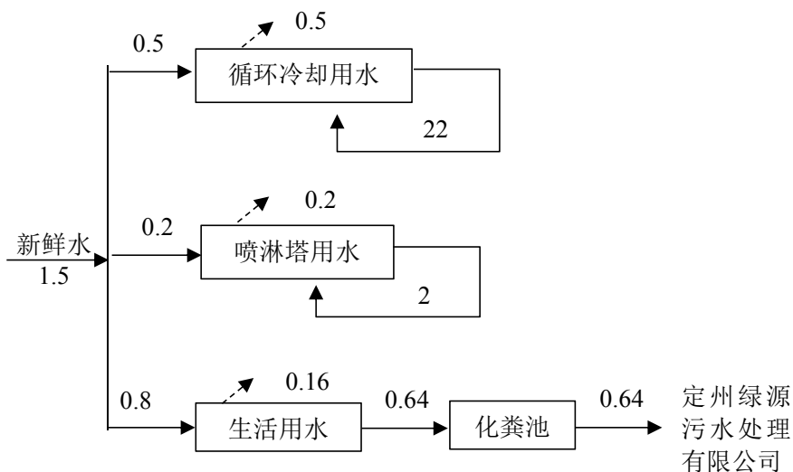
图 1 项目水平衡图 单位： \text{m}^3/\text{d}
