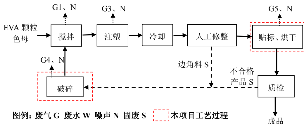
图 4 EVA 拖鞋生产工艺流程及污节点排图
