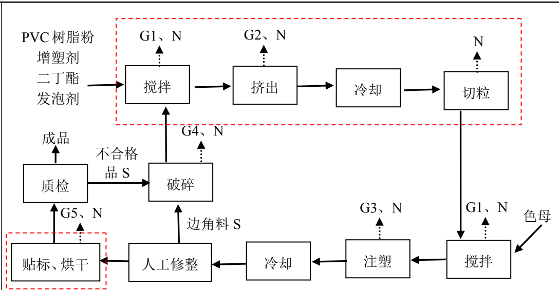
图例：废气 G 废水 W 噪声 N 固废 S 本项目工艺过程
