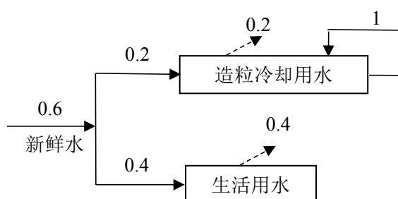
图 1 技改项目给排水平衡图 单位：m 3 /d
