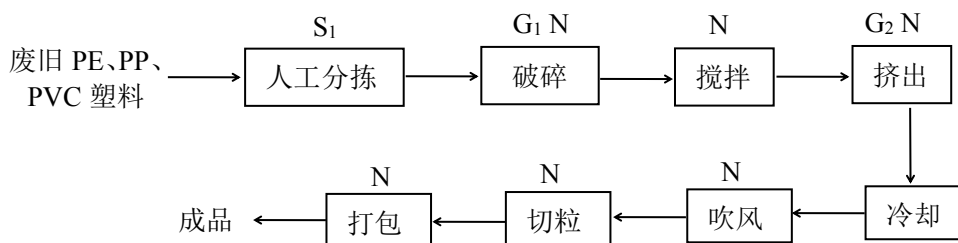
图 2 生产工艺流程及排污节点图
