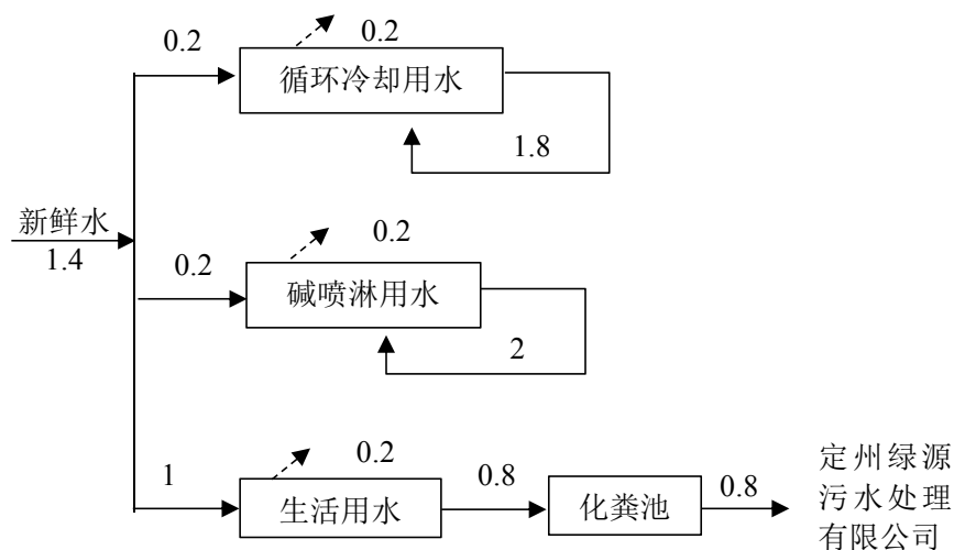
图 1 项目水平衡图 单位：m 3 /d
