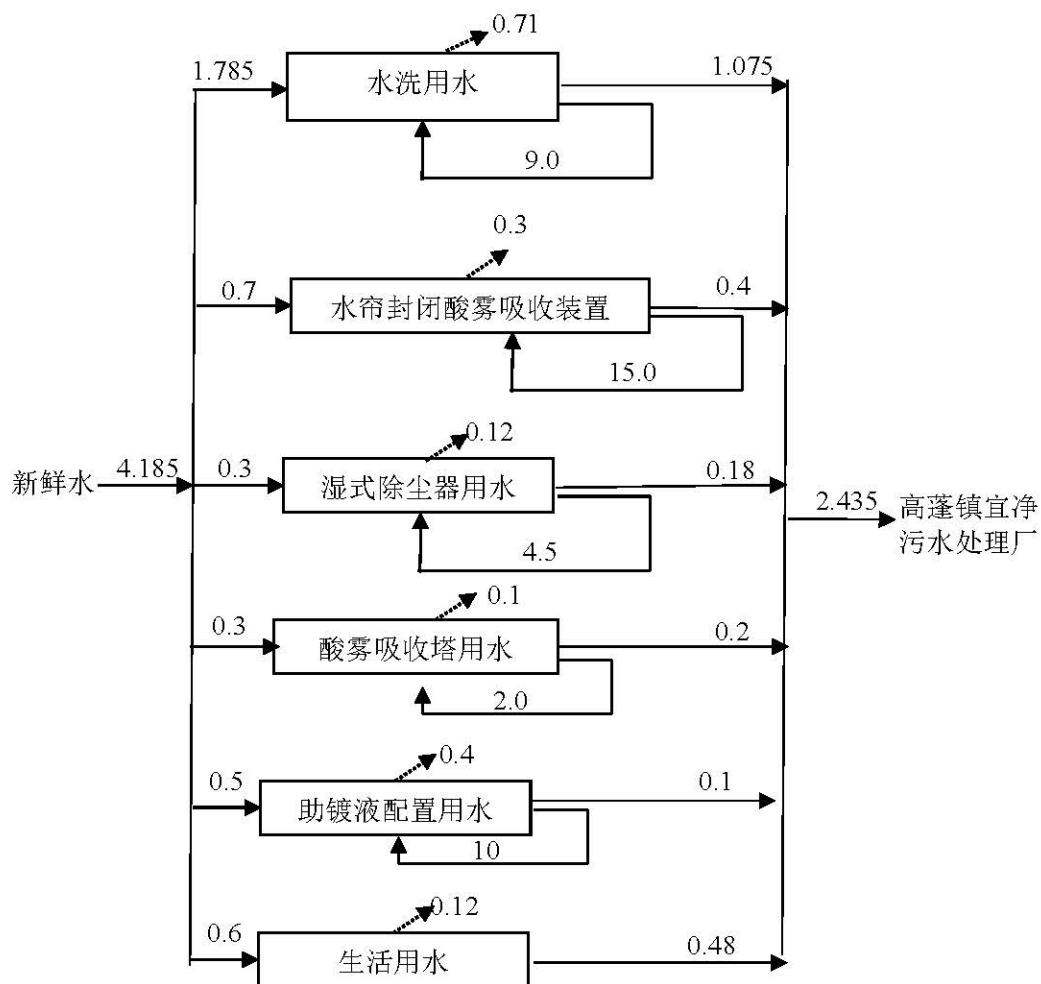
图 2 扩建后全厂水量平衡图 单位：m³/d
