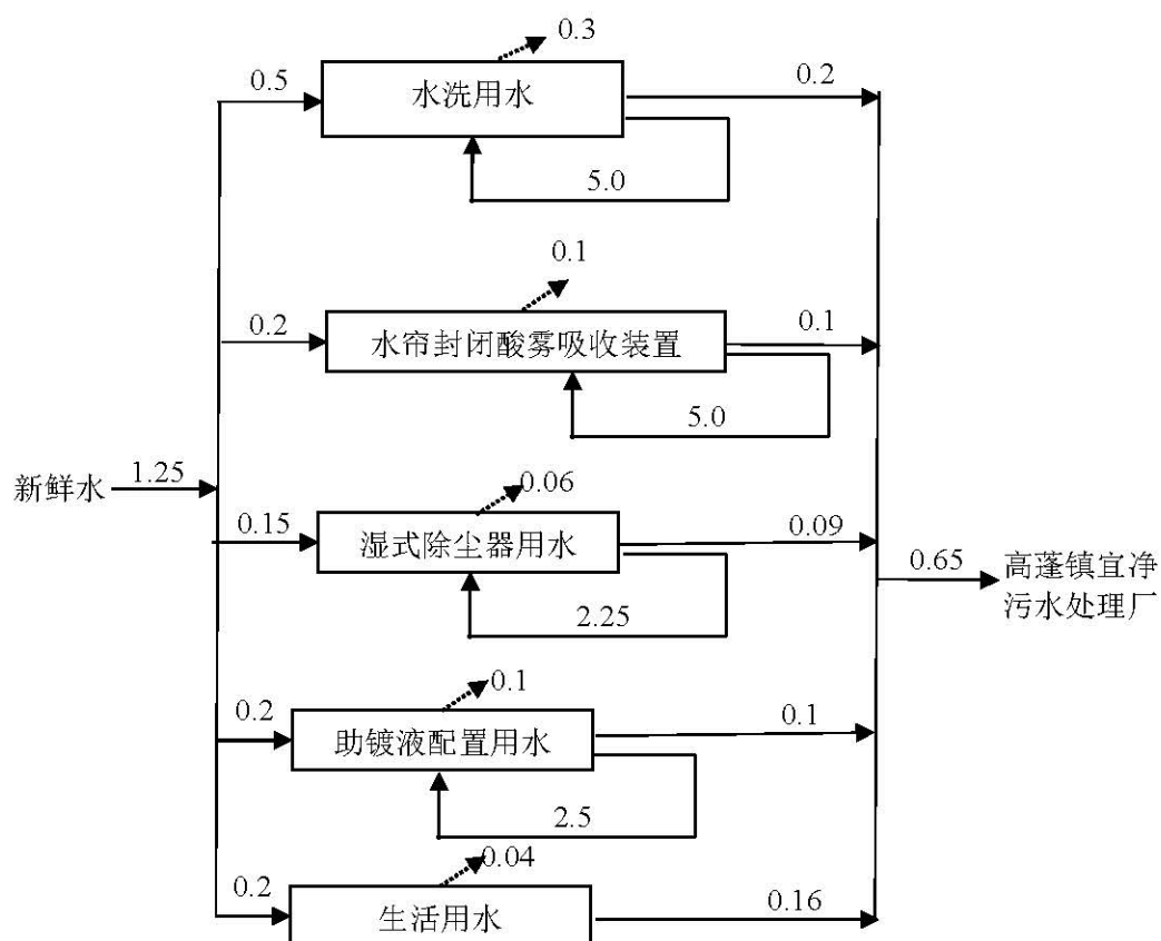
图 1 拟建项目水量平衡图 单位: \text{m}^3/\text{d}
