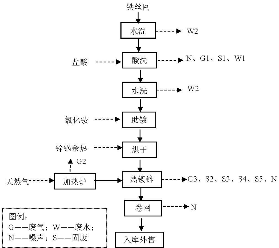
图 3 热镀锌网生产工艺流程及污节点排图
