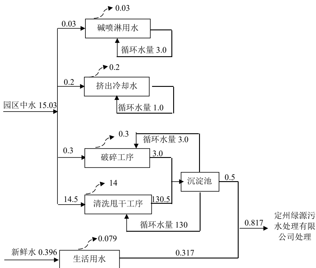
图 2.1 项目给排水平衡图 单位: \text{m}^3/\text{d}
