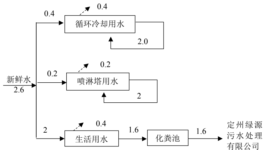
图 1 项目水平衡图 单位： \text{m}^3/\text{d}
