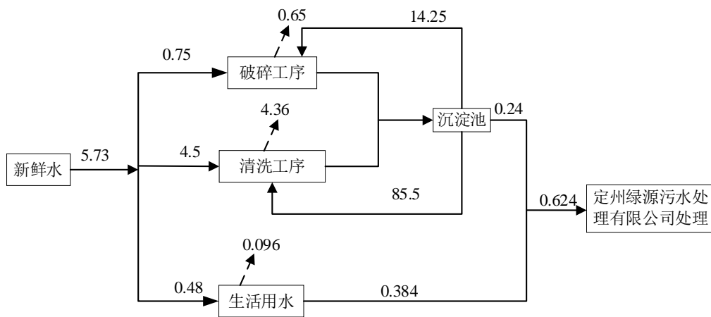
图1 本项目水平衡图 单位: m 3 /d
