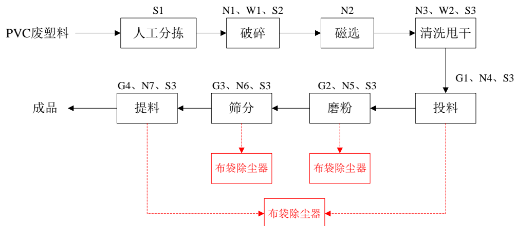
图2 项目生产工艺及产污节点图
