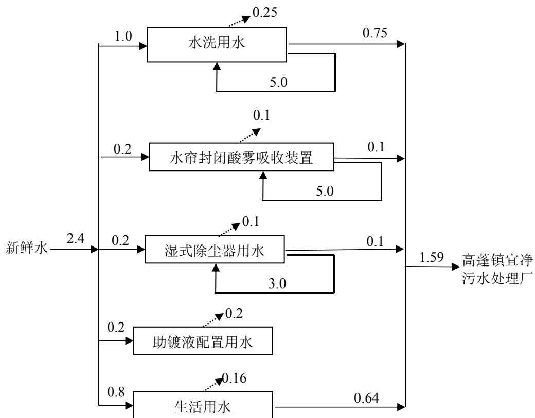
图 1 拟建项目水量平衡图 单位: \text{m}^3/\text{d}
