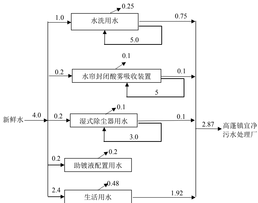
图2 全厂水量平衡图 单位: m 3 /d
