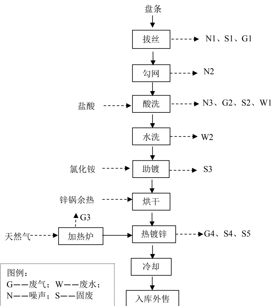
图 3 热镀锌丝生产工艺流程及污节点排图
