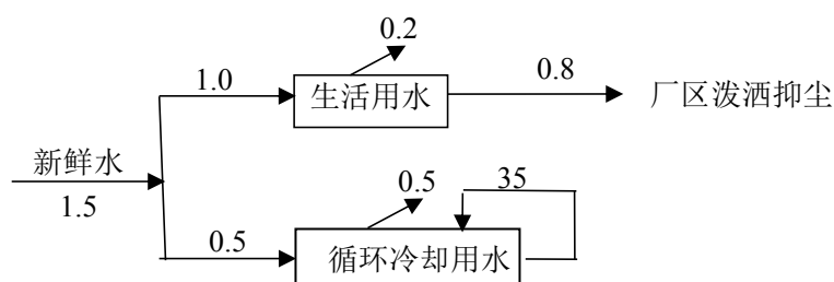
图 1 全厂项目给排水平衡图 单位：m 3 /d
