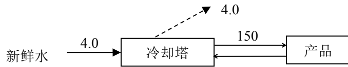
图 2-1 本项目给排水平衡图 (单位: m 3 /d)
