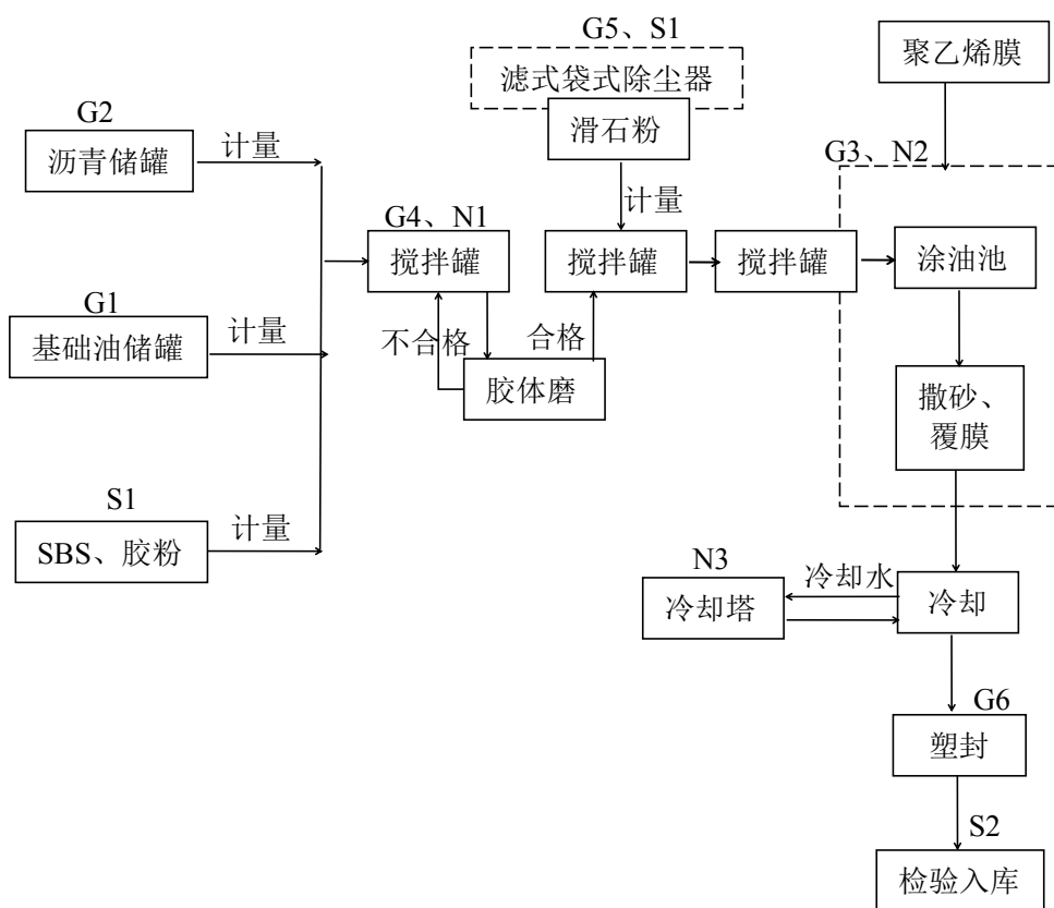
图 2-4 自粘防水卷材生产工艺流程及排污节点
