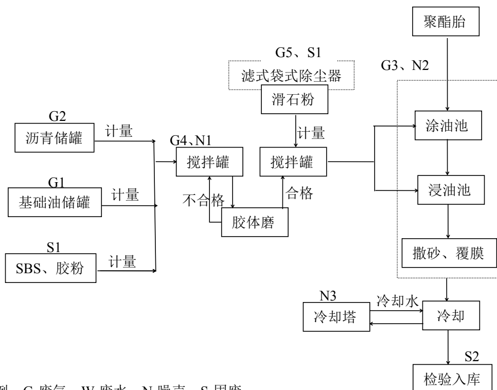
图 2-3 SBS 防水卷材生产工艺流程及排污节点
