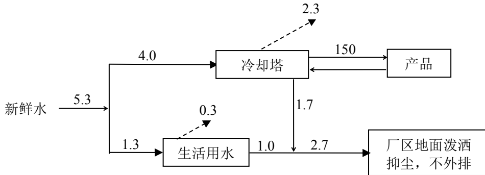
图 2-2 全厂给排水平衡图 (单位: m 3 /d)
