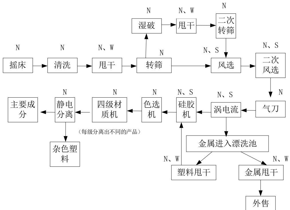
图2.2 废塑料破碎分选生产工艺及产污节点图
