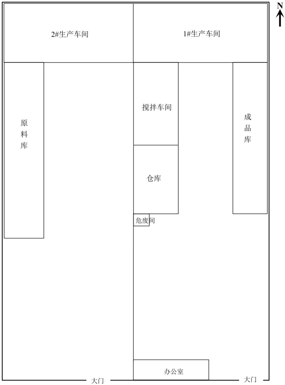
附图 3 建设项目总平面布置图
