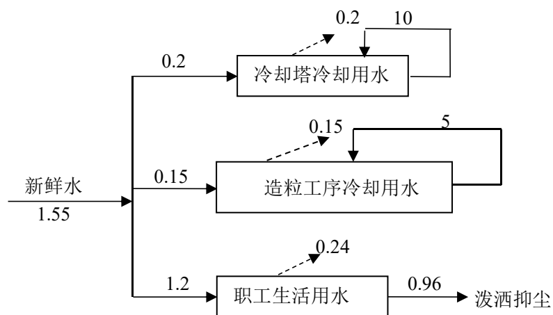
图 2-2 技改项目建成后全厂给排水平衡图 单位: \text{m}^3/\text{d}
