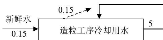
图 2-1 技改项目水量平衡图 单位： \text{m}^3/\text{d}
