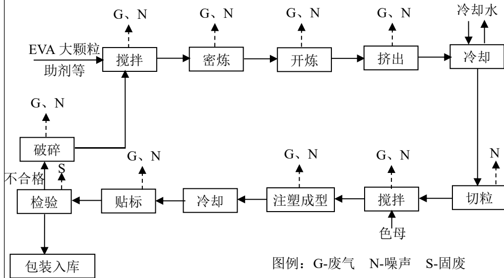
图 2-4 EVA 拖鞋生产工艺流程及产排污节点图
