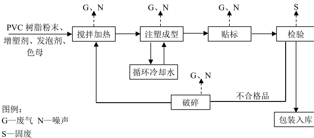
图 2-3 PVC 拖鞋生产工艺流程及排污节点图
