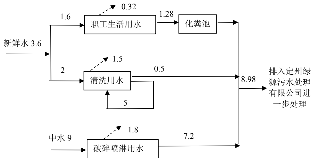
图1 项目给排水平衡图 单位：m 3 /d
