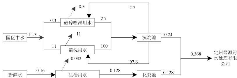
图2-1 项目给排水平衡图 单位：m 3 /d
