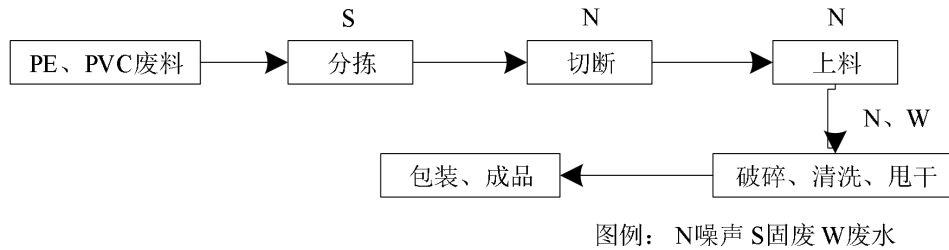
图 2-2 项目生产工艺及产污节点图
