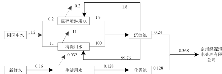
图2-1 项目给排水平衡图 单位：m 3 /d
