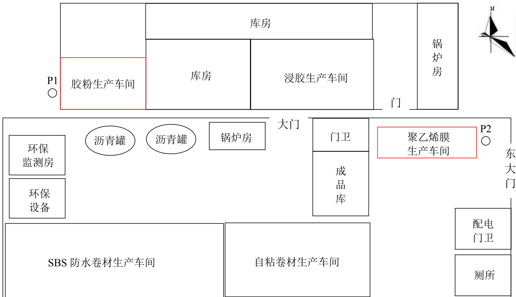
附图 3 项目平面布置图 比例: 1:200
