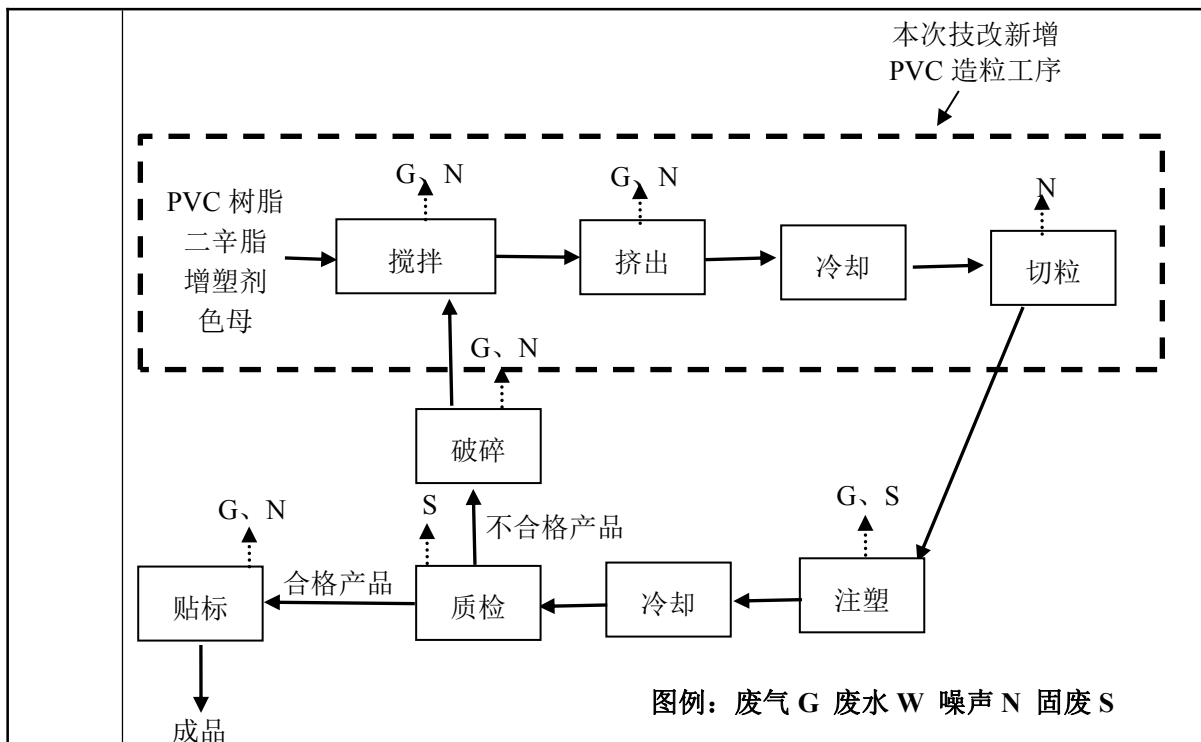
图 3 PVC 拖鞋生产工艺流程及排污节点排图
