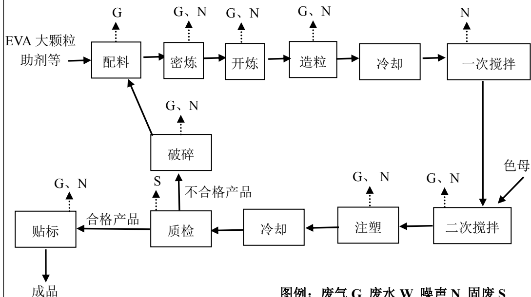
图 4 EVA 拖鞋生产工艺流程及污节点排图
