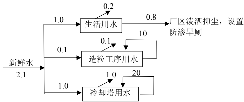
图 2 技改后全厂项目给排水平衡图 单位: \text{m}^3/\text{d}
