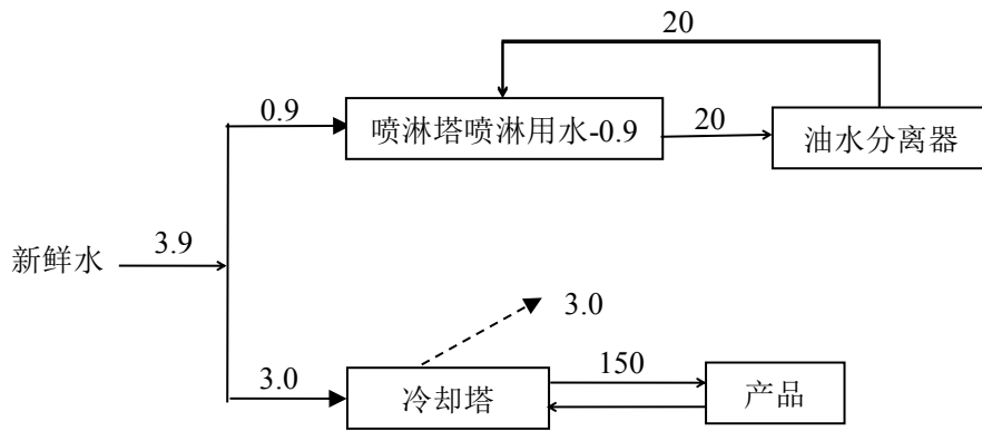
图 2-1 本项目给排水平衡图（单位： \text{m}^3/\text{d} ）
