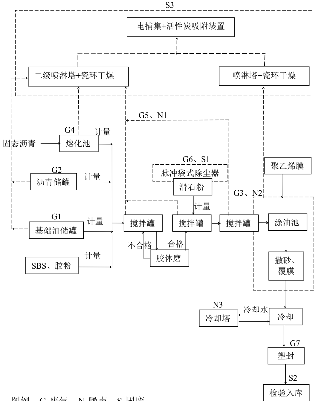
图 2-3 自粘防水卷材生产工艺流程及排污节点
