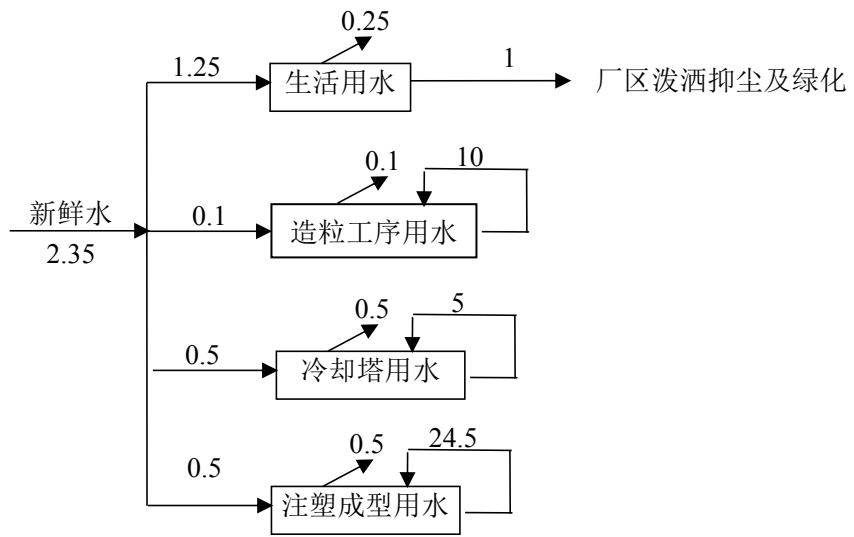
图2 技改后全厂项目给排水平衡图 单位：m 3 /d
