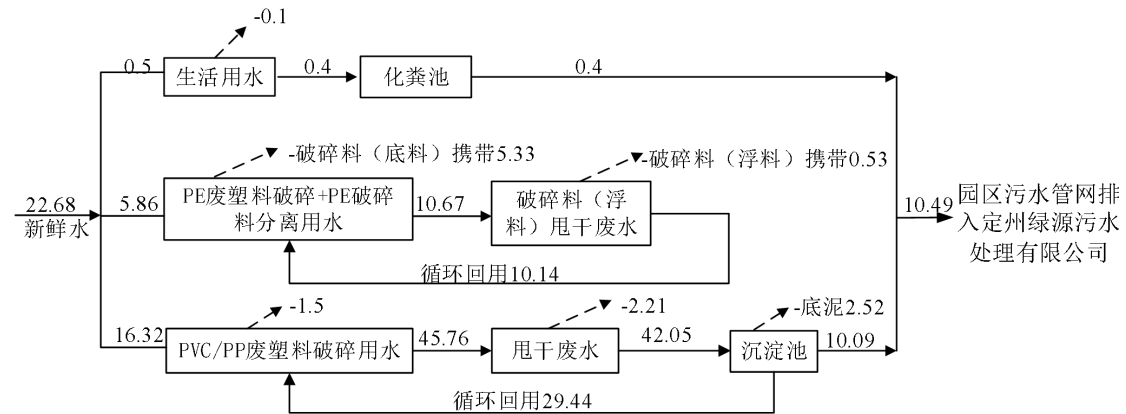
图 1 给排水平衡图 单位：m 3 /d
