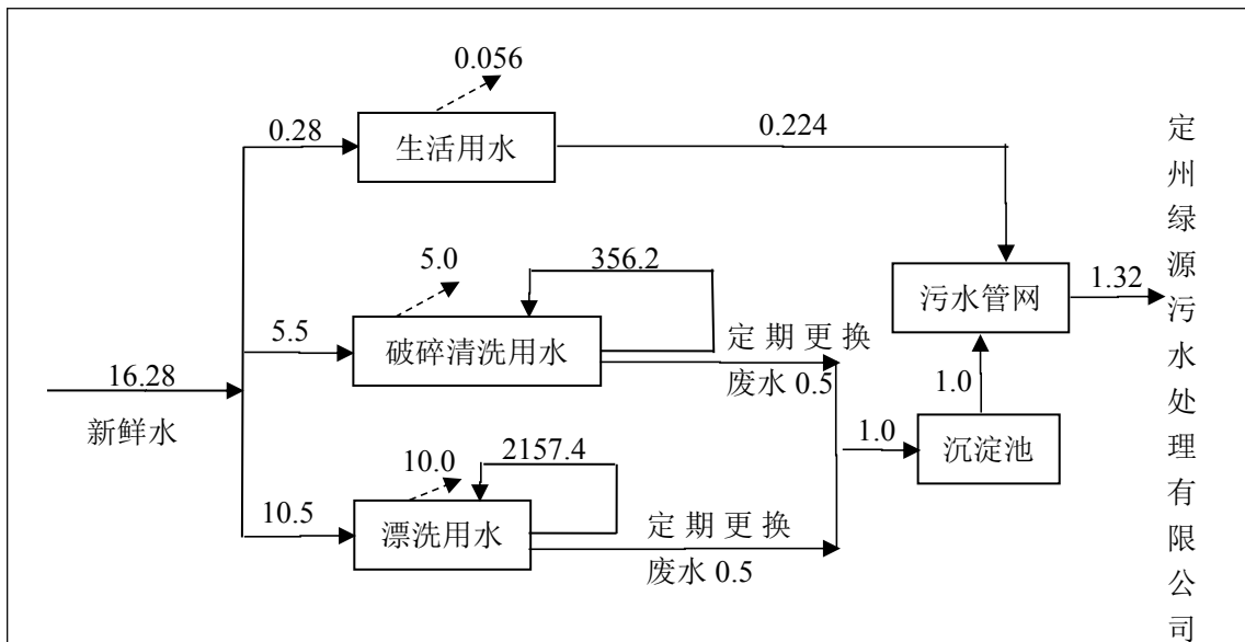
图 1 项目水量平衡图 单位: m 3 /d
