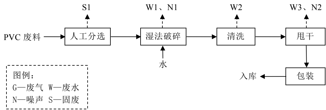
图 2 项目生产工艺流程图
