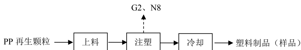
图 3.2-2 注塑生产工艺流程图
