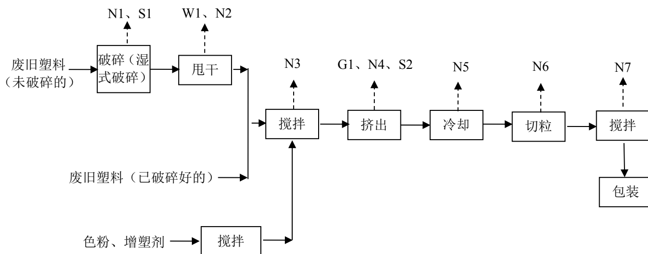
图 3.2-1 造粒生产工艺流程图
