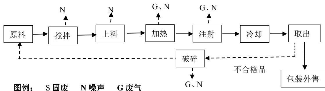
图2 产品原料工艺流程及排污节点图
