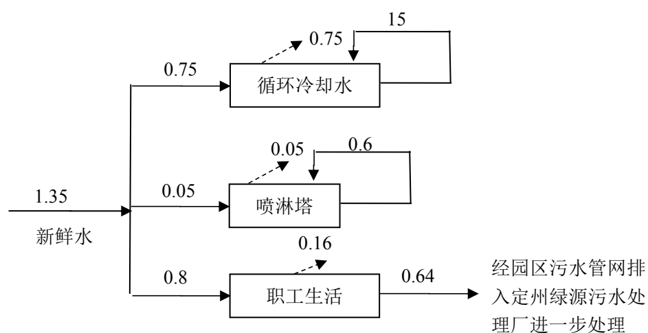
图 1 项目水量平衡图 单位： \text{m}^3/\text{d}
