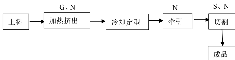
图 2 产品原料工艺流程及排污节点图
