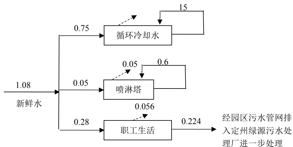
图 1 项目水量平衡图 单位：m³/d
