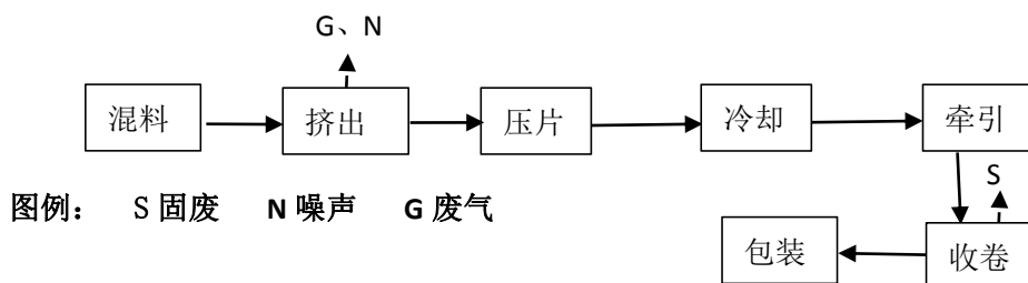
图 4 EVA 板材工艺流程及排污节点图
