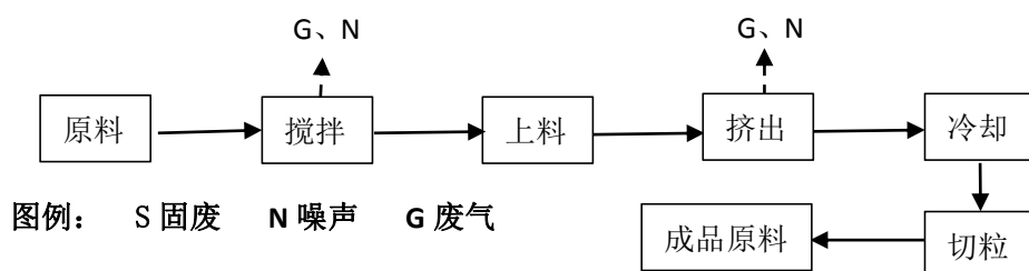
图 2 产品原料工艺流程及排污节点图
