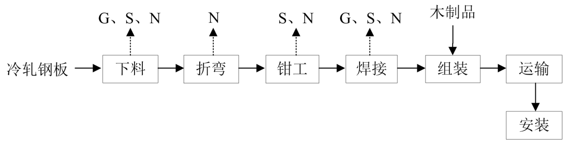
图2 生产工艺流程及产污节点图
