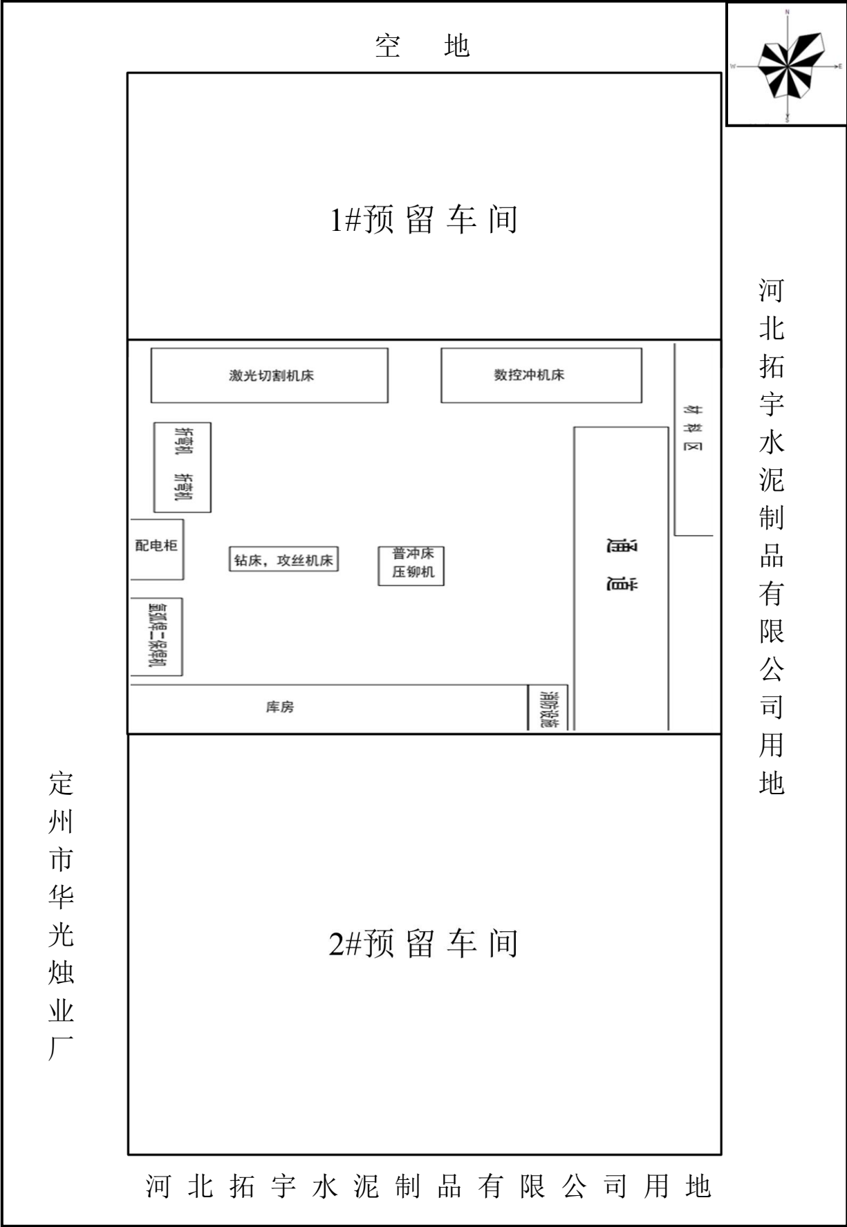
附图3 项目平面布置及周边关系图
