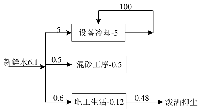
图 2 水平衡图 单位: \text{m}^3/\text{d}
