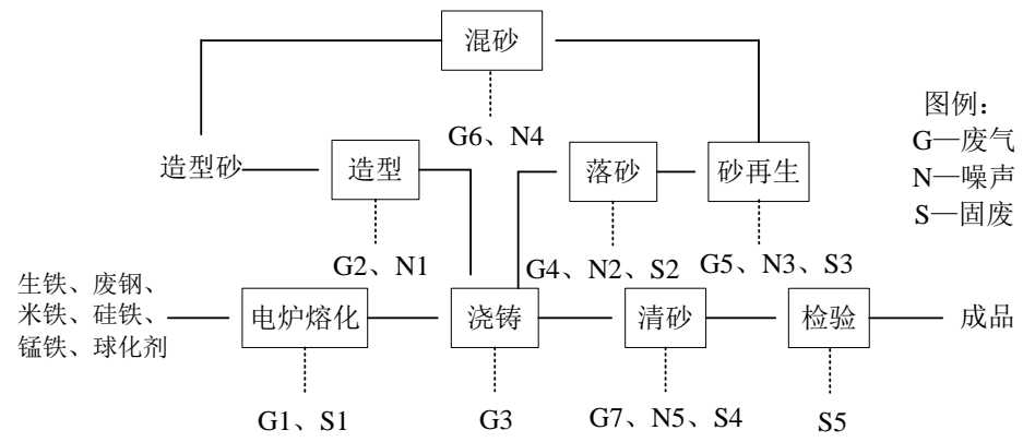
图 4 生产工艺流程及排污节点图
