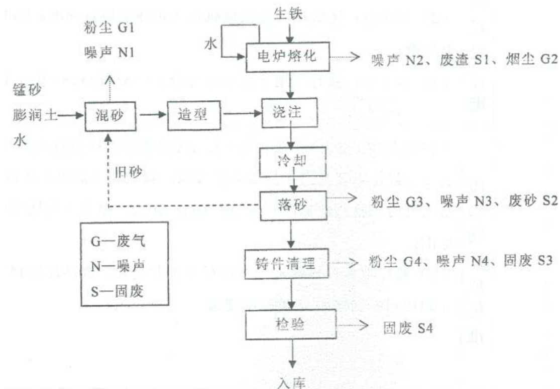
图1 生产流程及排污节点
