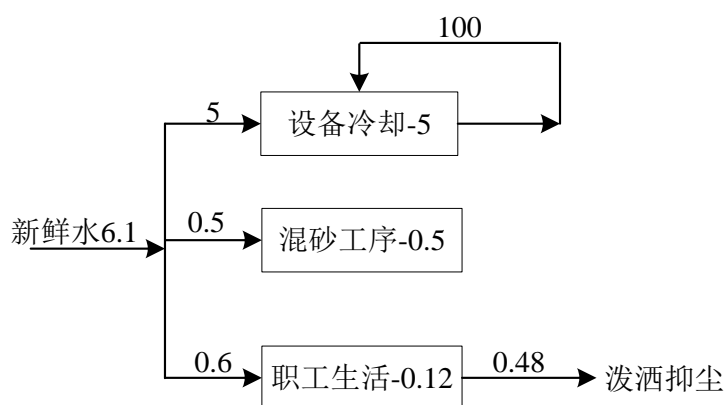
图 3 水平衡图 单位：m³/d
