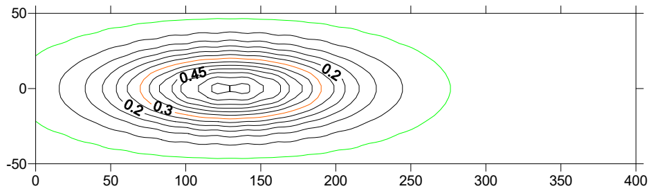
图 6 石油类污染运移 1000d
