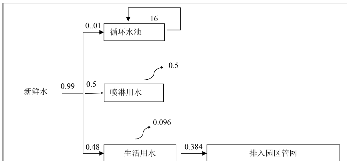
图1 本项目水平衡图（单位：m³/d）
