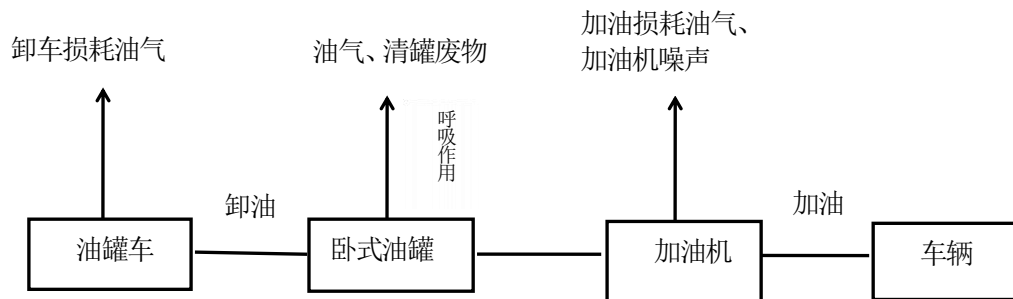
图 2 成品油销售总工艺流程图
