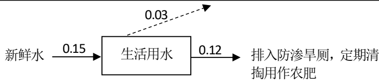
图1 项目水平衡图（单位：m 3 /d）
