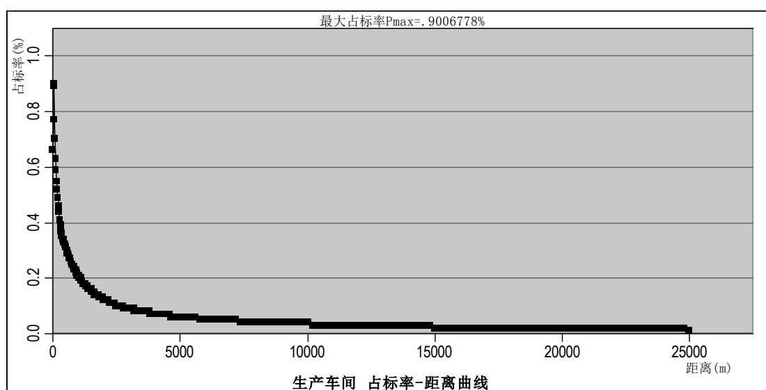
图 5.2-3 面源（生产车间）最大 P_{\max} 和 D_{10\%} 预测结果图
