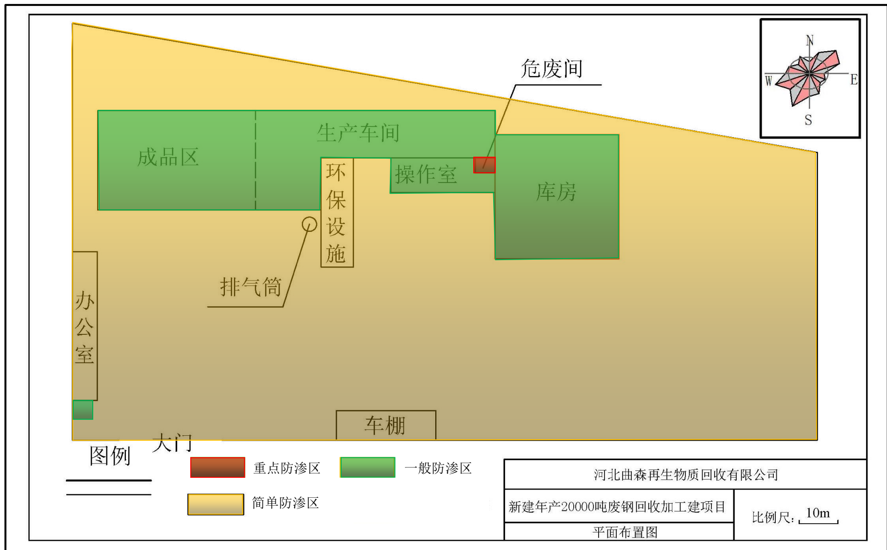
附图 8 项目厂区分区防渗图
