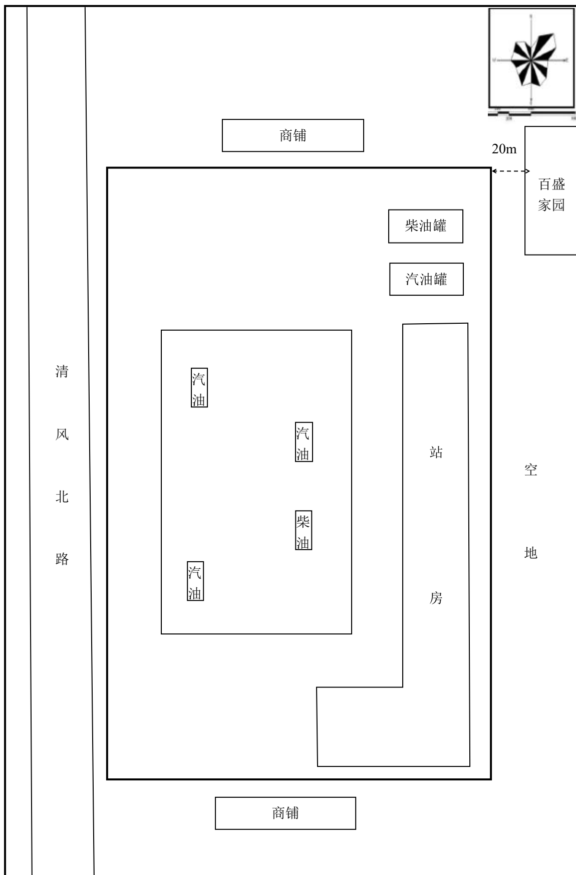
附图 3 项目周边关系及平面布置图
