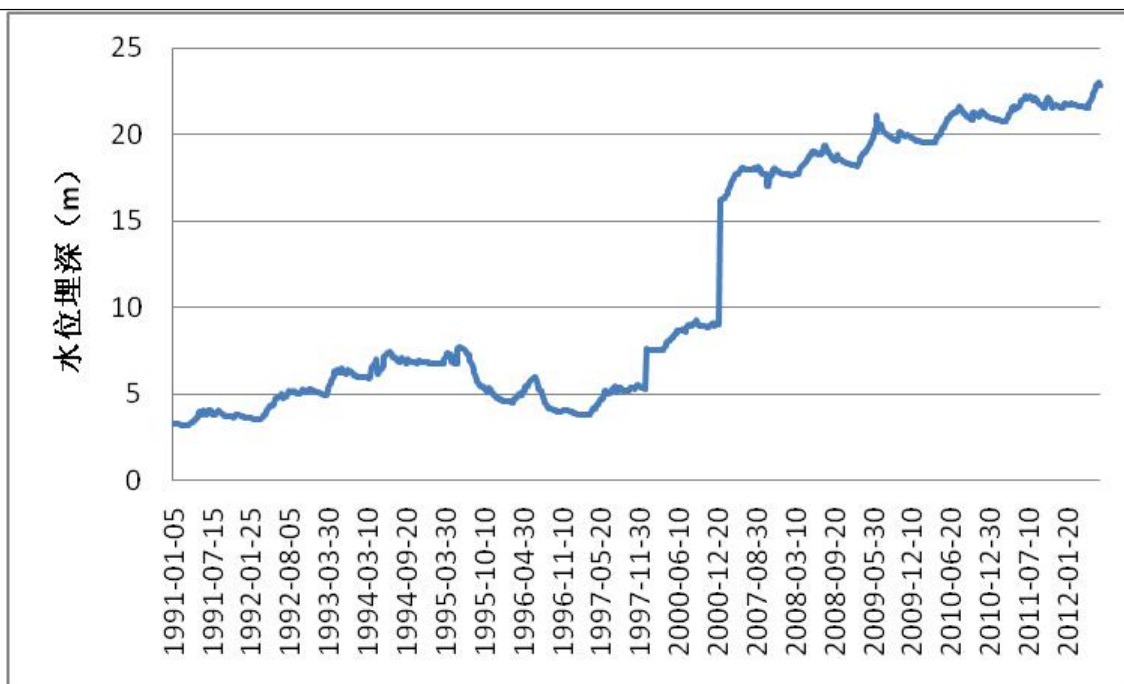
图 13 西城乡支白土村北地下水监测点水位动态曲线
