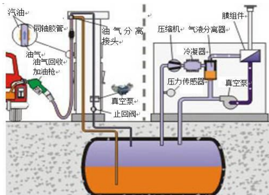
图 7 油气排放装置示意图
