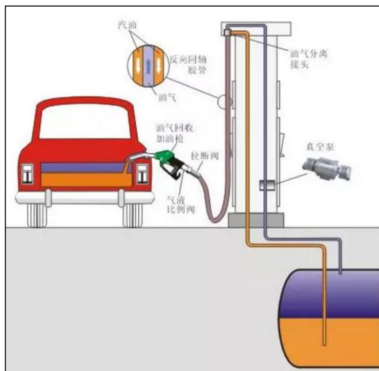
图5 分散式二次油气回收系统示意图
