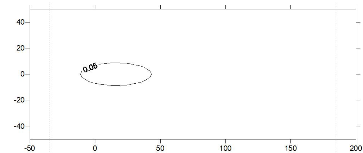
图 14 含水层中污染晕影响范围图
