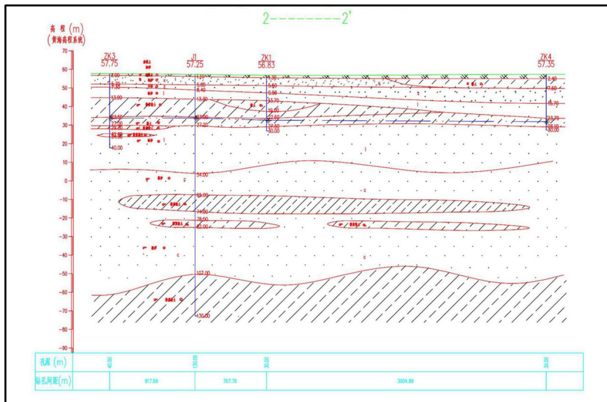
图 12 2—2'水文地质剖面图
