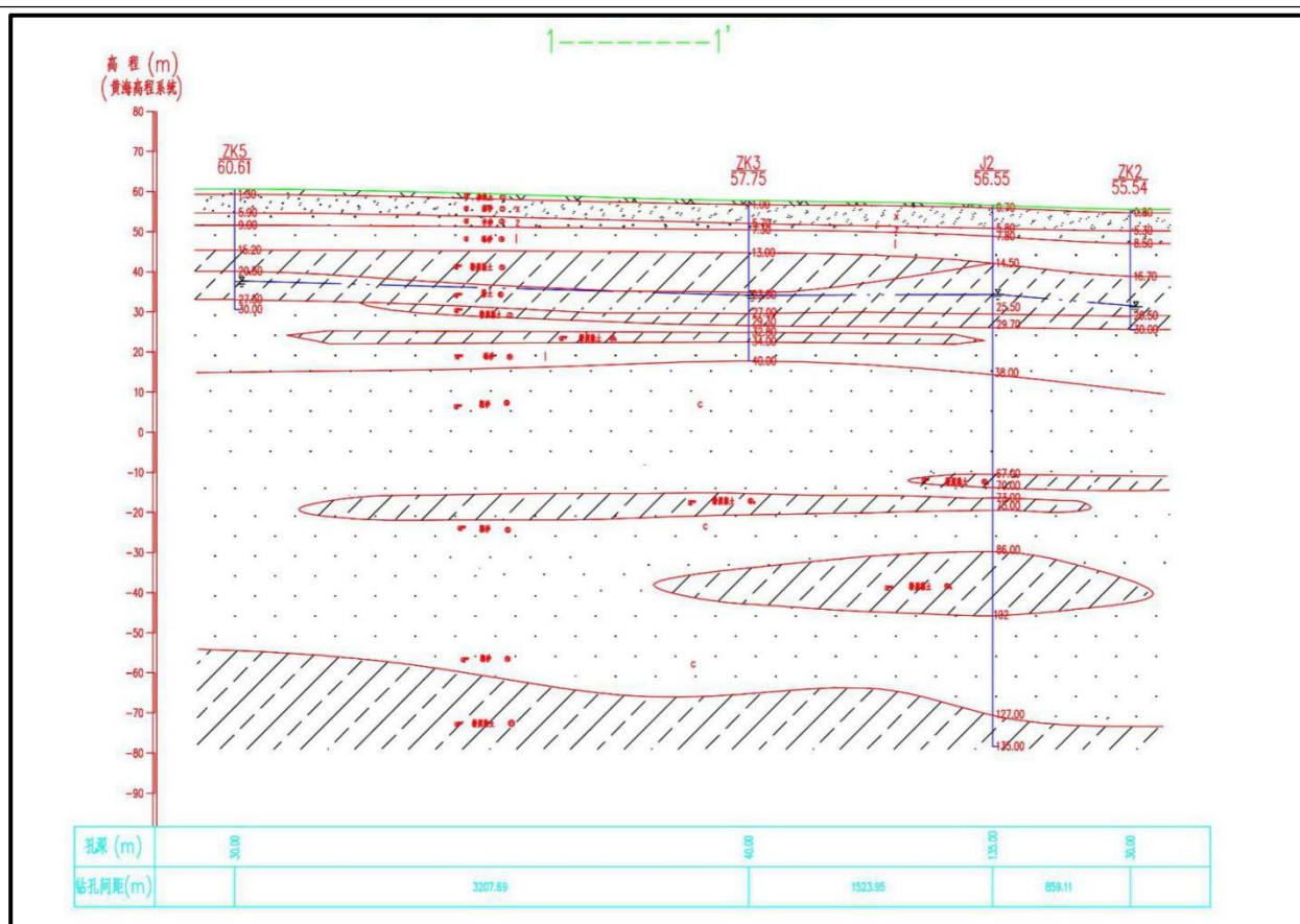
图 11 I—I'水文地质剖面图
