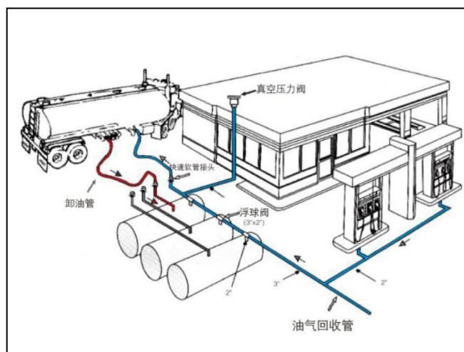
图4 一次油气回收示意图
