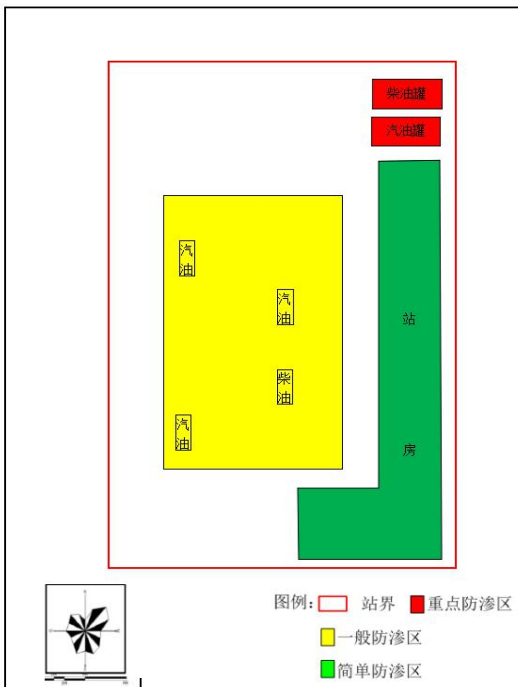
图 15 项目分区防渗布置图
