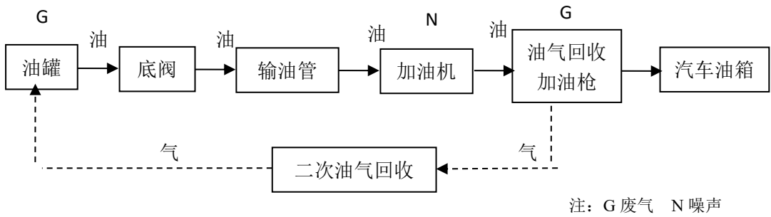
图 3 加油工艺流程及排污节点
