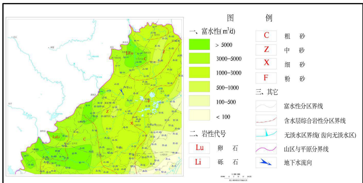
图10 区域水文地质图
