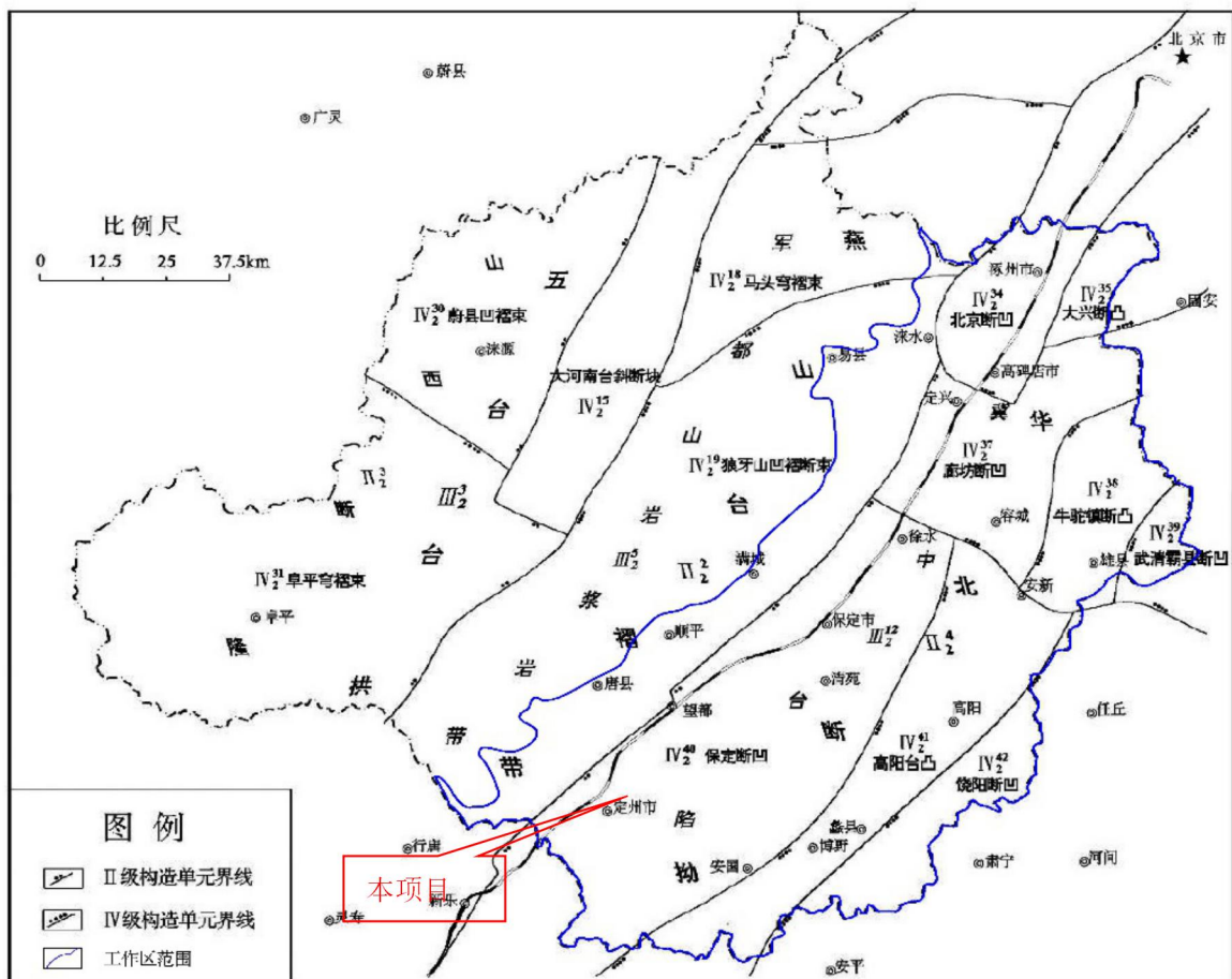
图9 保定地区构造单元分区图
