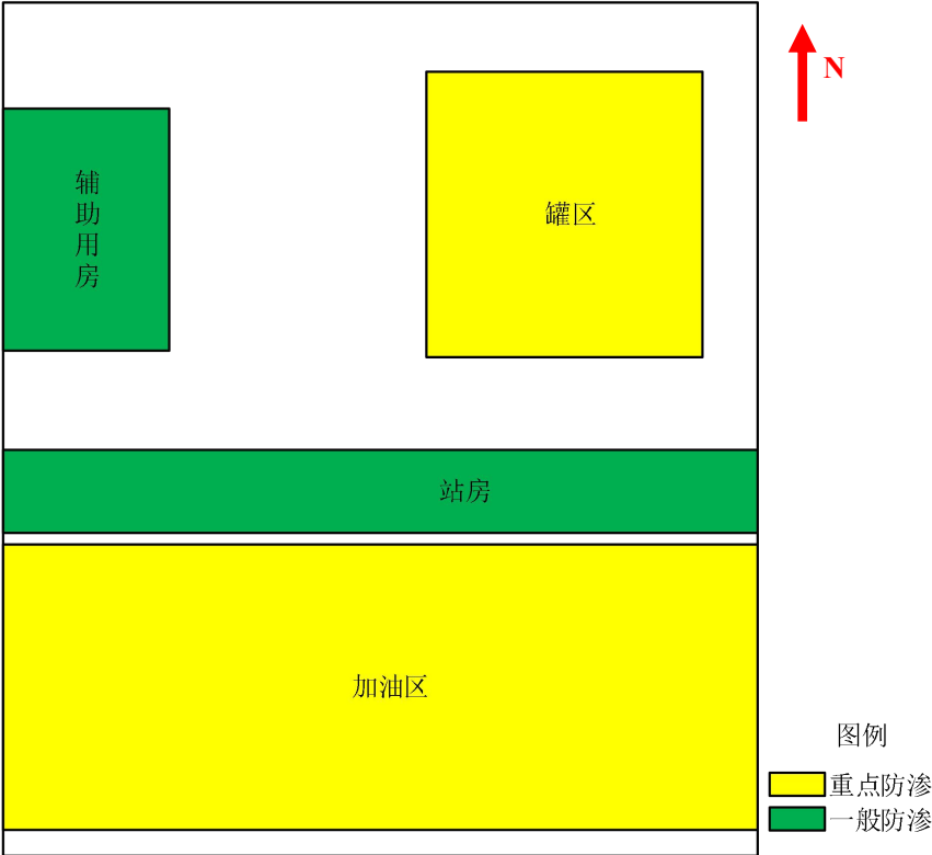
图 8 防渗分区图
