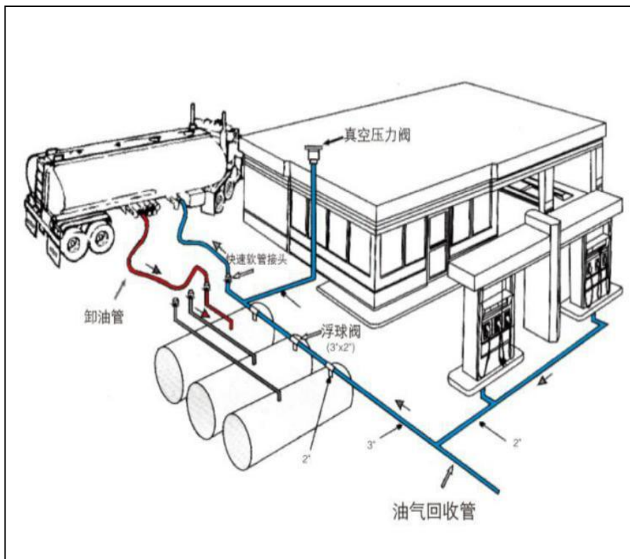
图5 一次油气回收示意图
