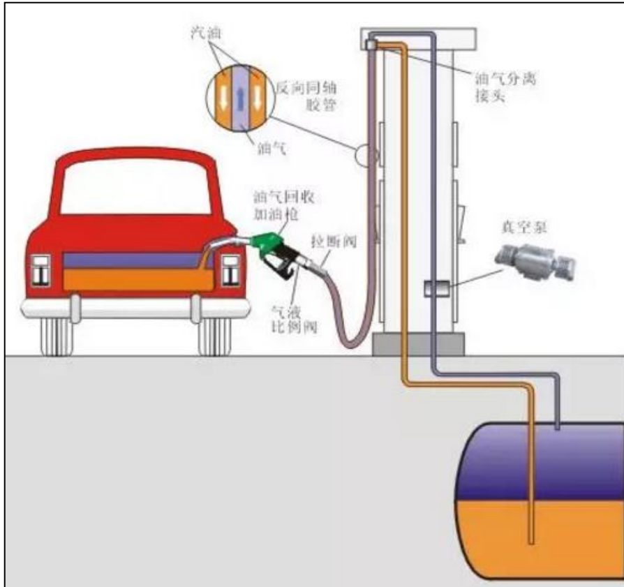
图 6 分散式二次油气回收系统示意图
