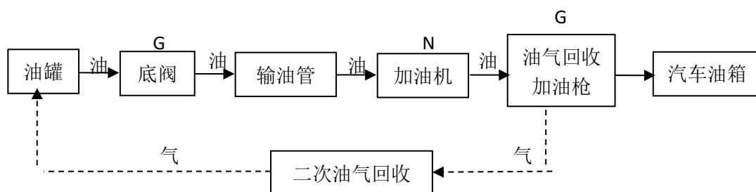
图 4 加油工艺流程及排污节点
