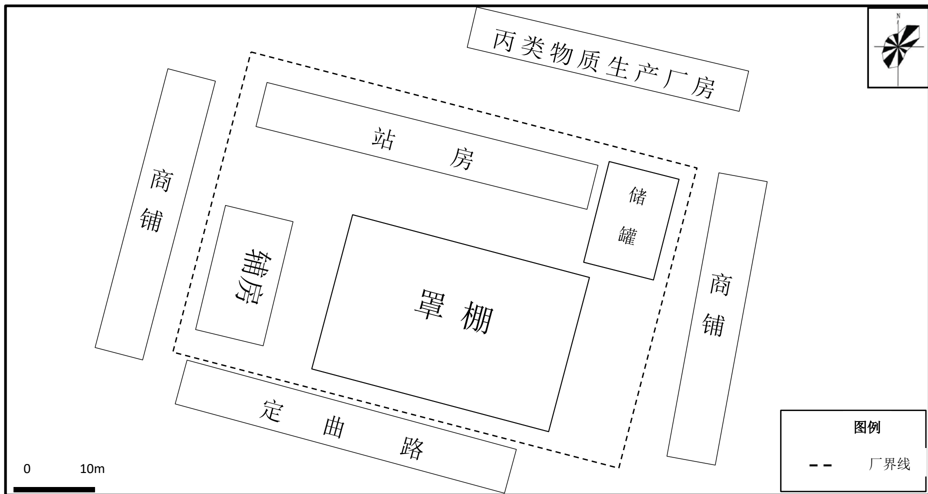
图3 厂区平面布置图
