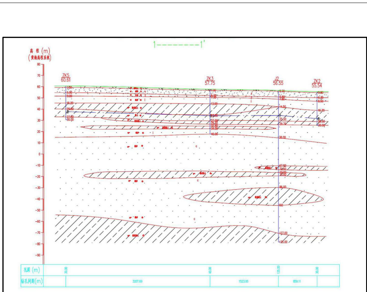
图 10 I—I'水文地质剖面图
